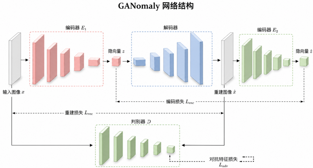
图 1 GANomaly 网络结构示意图
