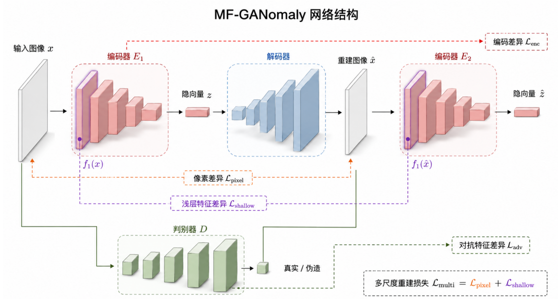
图 2 MF-GANomaly 网络结构示意图
