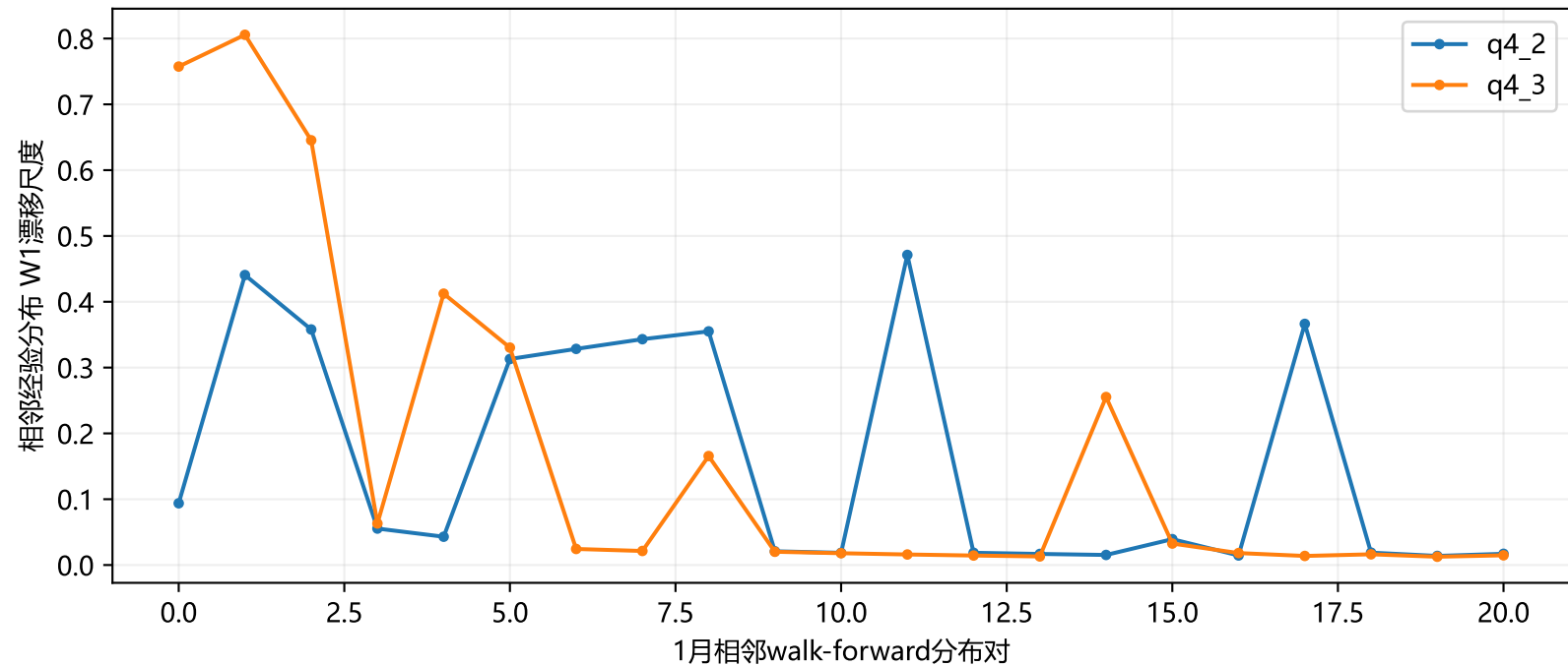
附图B \epsilon 校准：经验分布漂移尺度（非置信半径）
