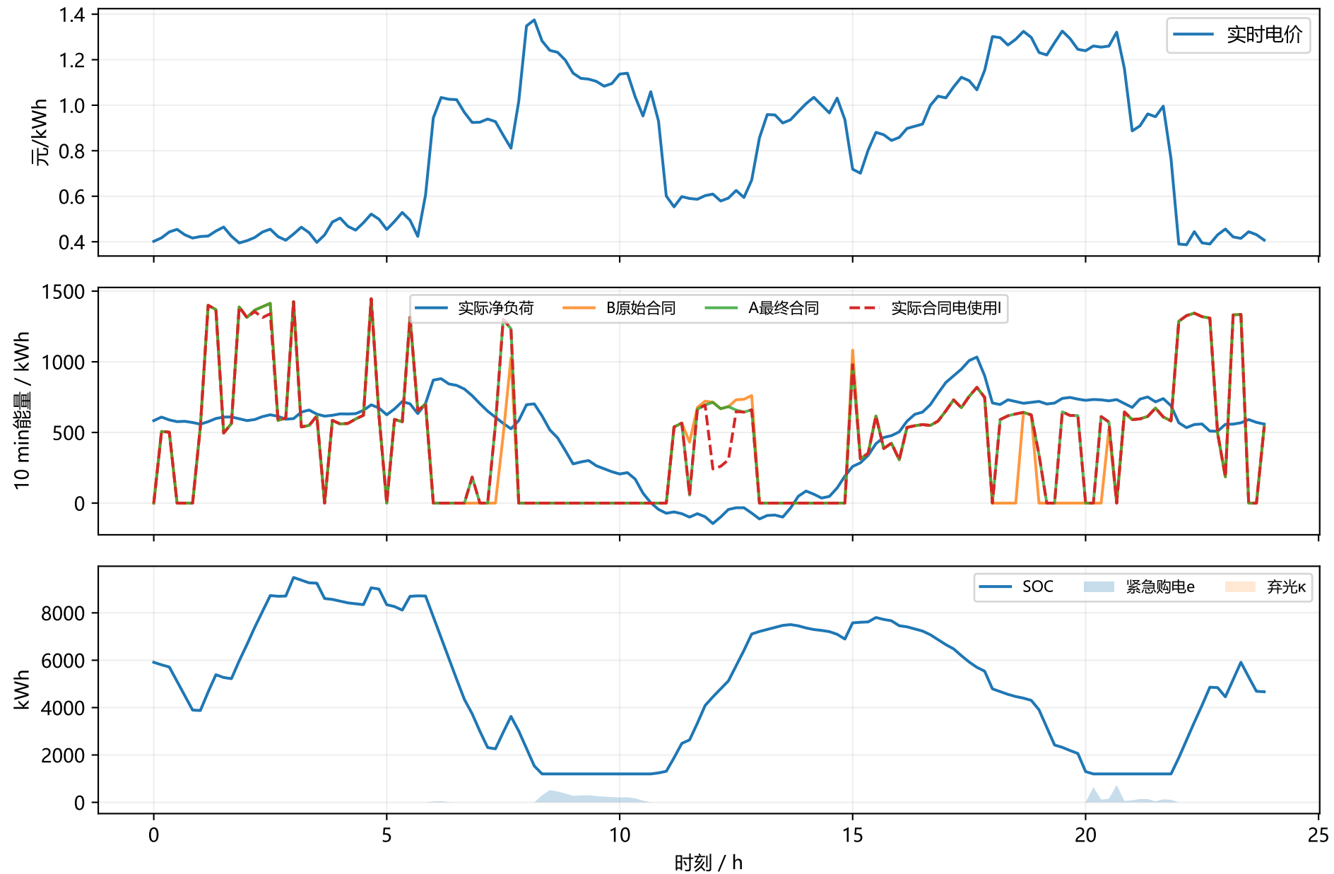
图5 Q4-3典型高成本日联合调度：2025-02-23（接近日费用95%分位）
