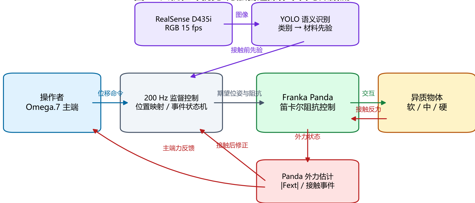
图 1 人机在环视觉-力融合遥操作平台与数据流
