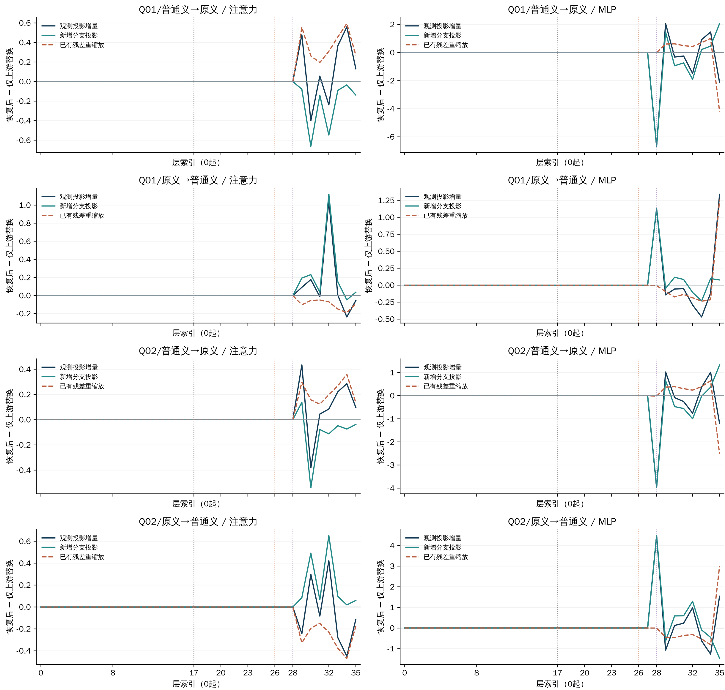
restore-L28-mlp : 全部36层增量及RMS分解 (非独立因果份额)
