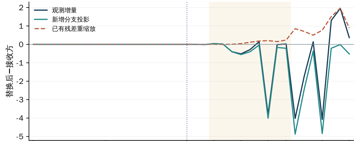
Q02 / 原义→普通义 / 注意力子层
