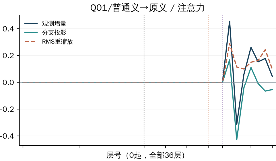
已有26注意力恢复后，再恢复28MLP：AB—A；答案前位置，原始投影的差值，非独立因果份额
