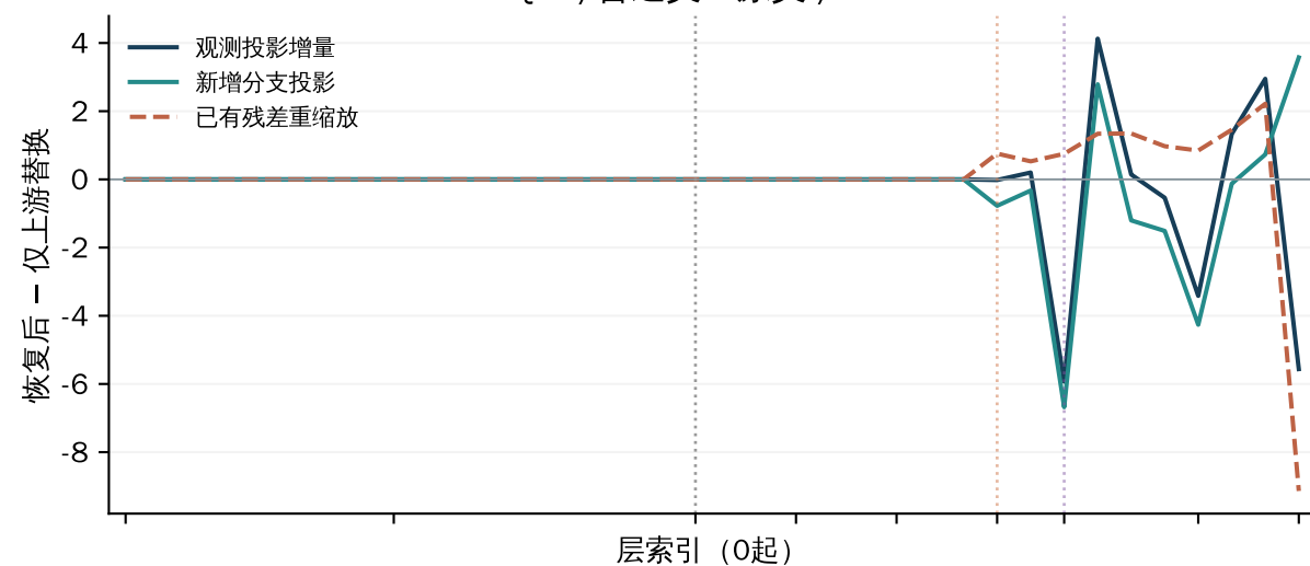
Q01/原义→普通义 / MLP
