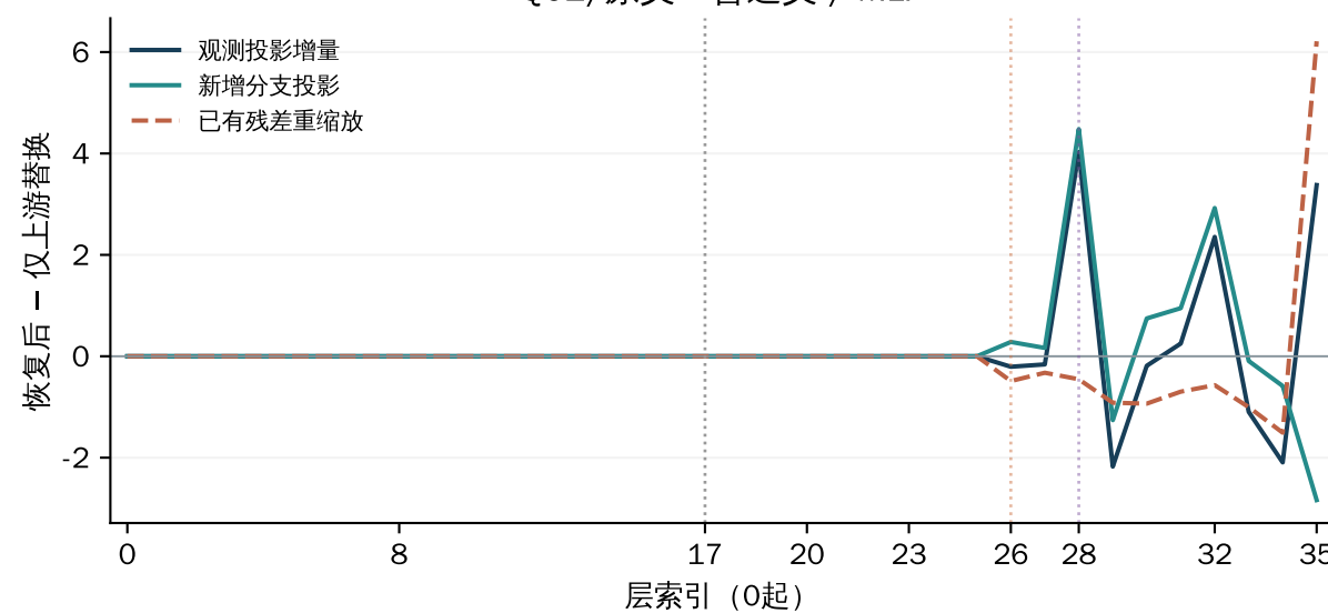
Q02/原义→普通义 / MLP
