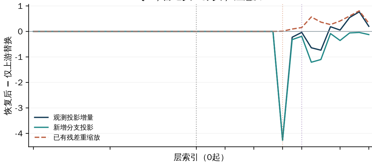
Q02/原义→普通义 / 注意力
