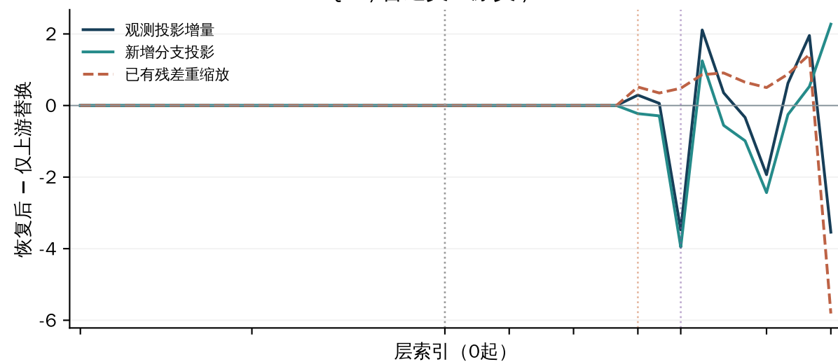
Q02/原义→普通义 / MLP
