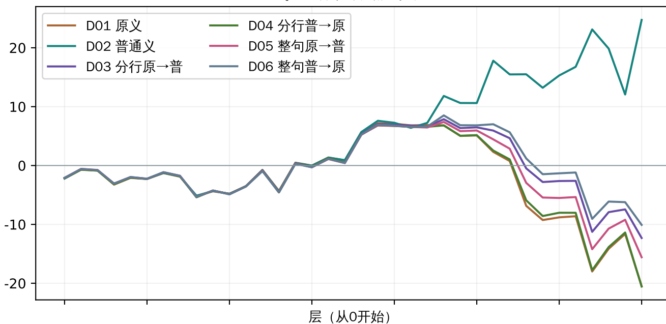
Q02 · 答案前块输出投影
