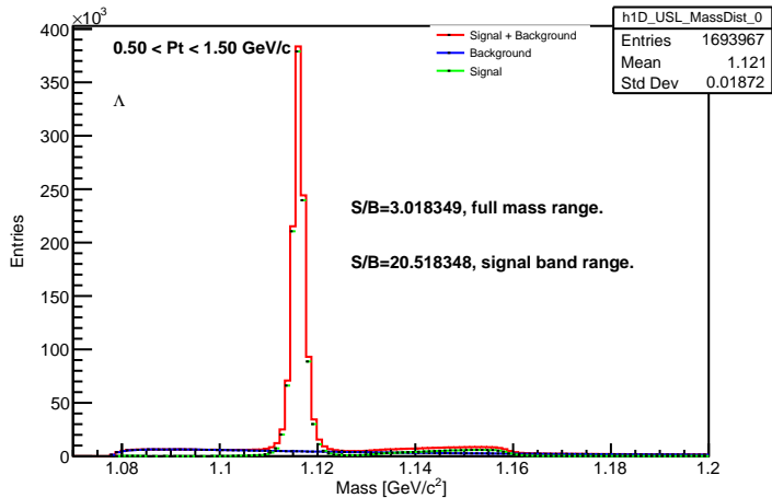
h1D_USL_MassDist_0
