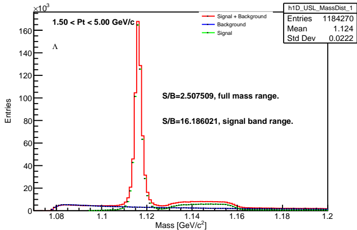
h1D_USL_MassDist_1
