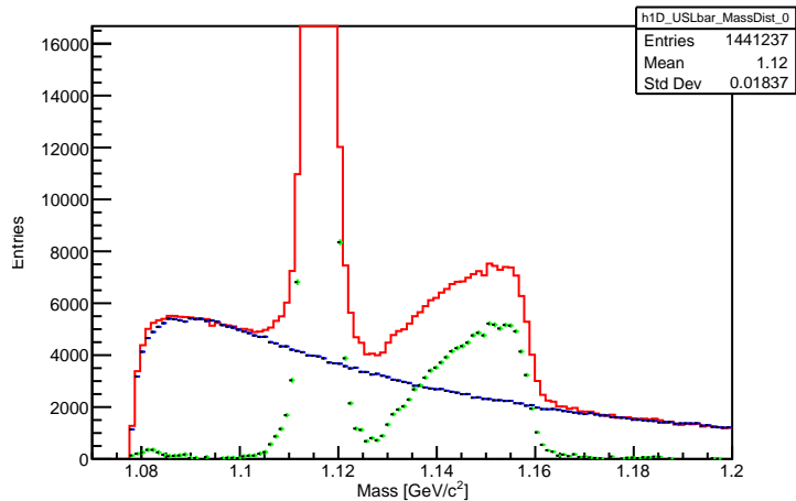
h1D_USLbar_MassDist_0
