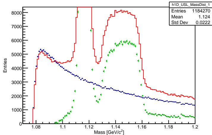
h1D_USL_MassDist_1
