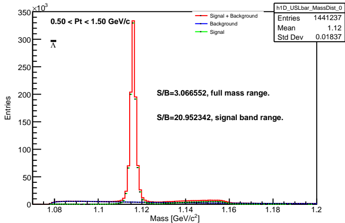
h1D_USLbar_MassDist_0
