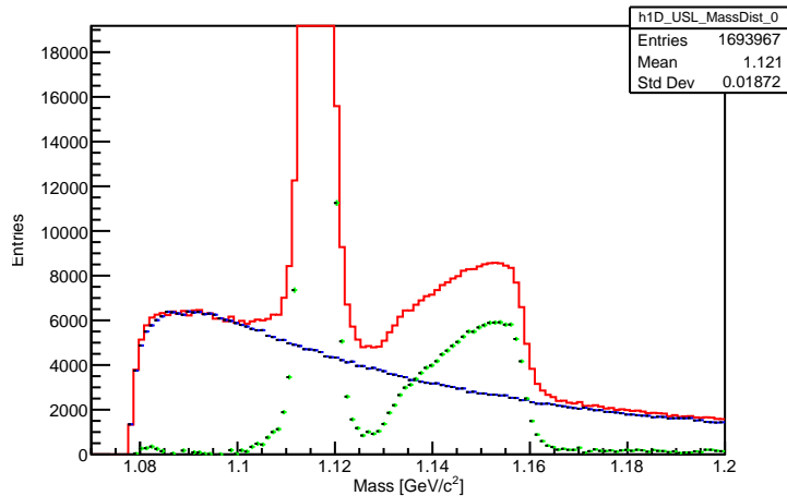
h1D_USL_MassDist_0
