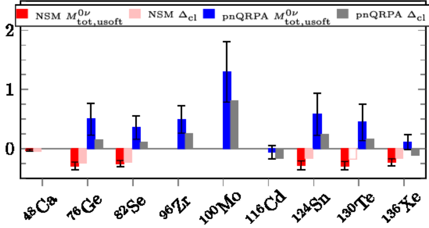
图 7: Total ultrasoft NME 与 non-closure correction 的比较 (参考自文献 [?])。二者量级相近, 说明 \text{N}^2\text{LO} ultrasoft 项不是形式上的小修正。
