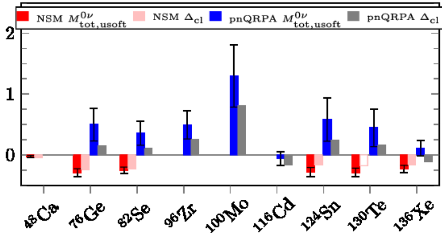
图 7: Total ultrasoft NME 与 non-closure correction 的比较（参考自文献 [4]）。二者量级相近，说明 N^2LO ultrasoft 项不是形式上的小修正。
