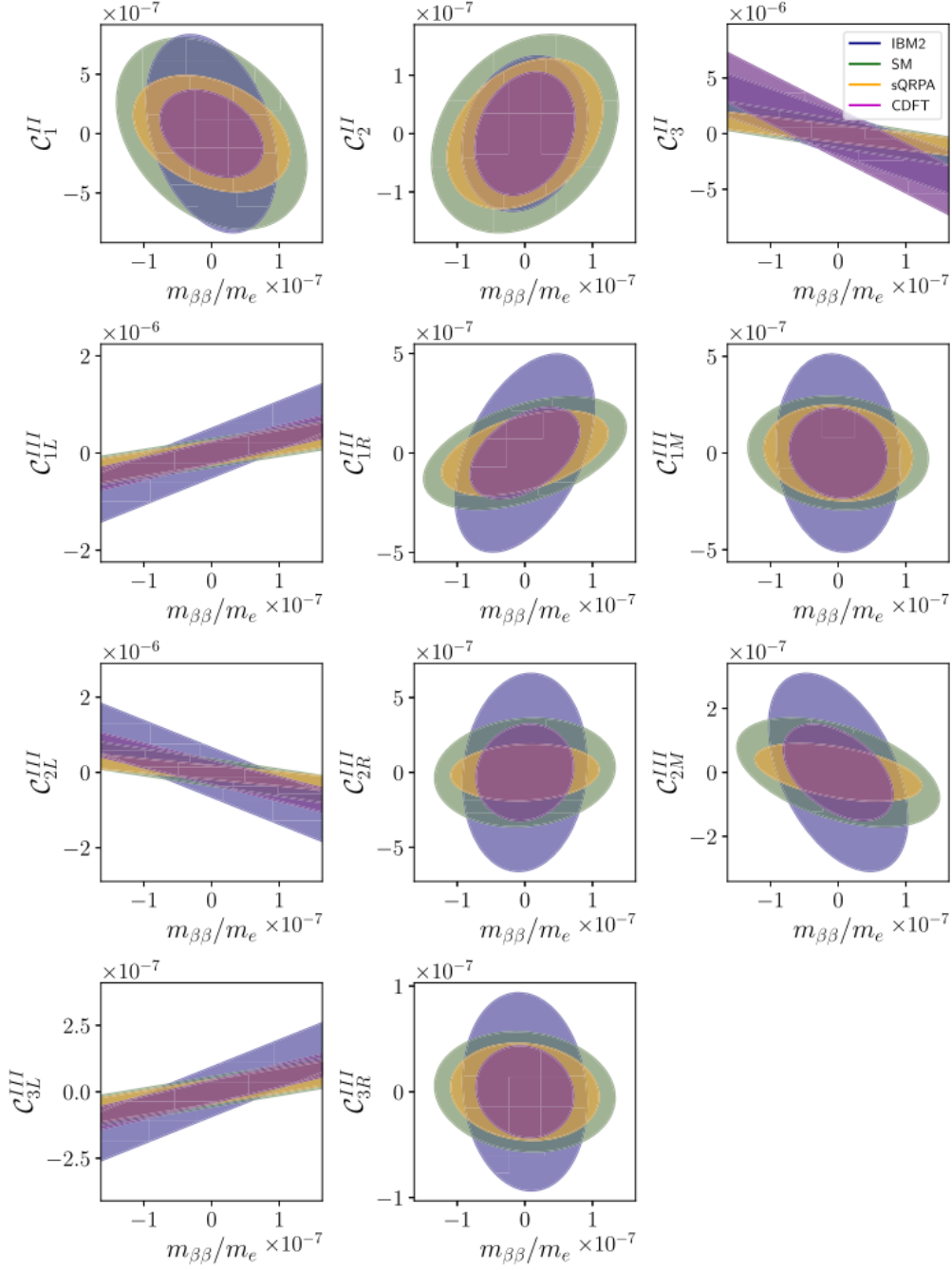
图 12: 文献 [5] LNV 系数之间的相关性分析。
