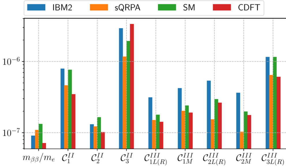
图 11: 文献 [5] 不同核模型对 LNV 系数的约束比较。
