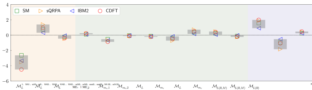
图 10: 文献 [5] 不同核模型对 ^{136}\text{Xe} 的组合 NME 比较。
