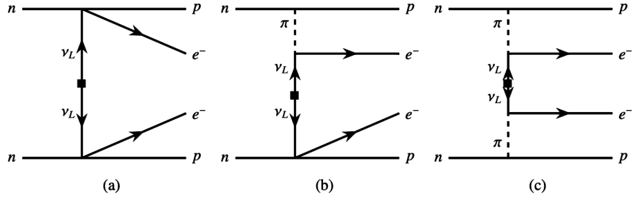
(a) Type-I: 标准轻 Majorana 中微子交换机制 [5]
