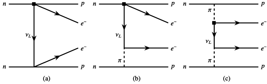
(b) Type-II: 长程非标准机制 [5]
