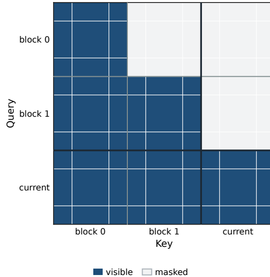
图 3: BELF 一次前向的注意力。查询看行、键看列。
