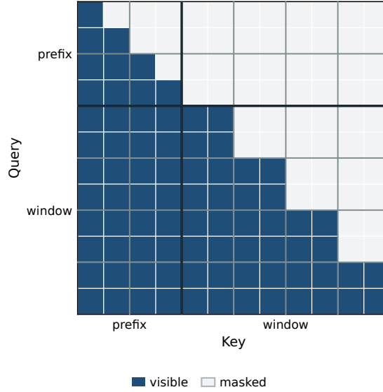
图 7: RELF 一次前向的注意力。查询看行、键看列。
