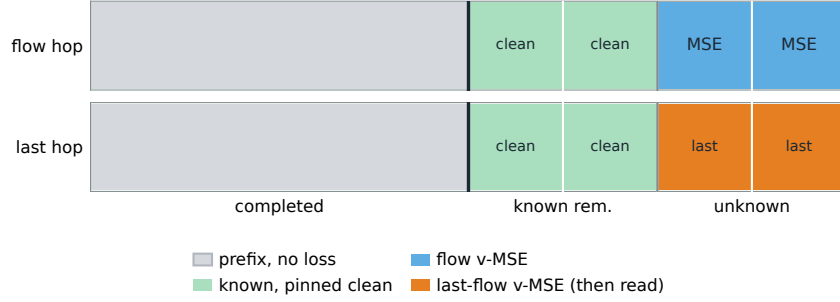
图 1: BELF clean: 当前块左侧为已知余数，钉干净、不进损失；右侧未知槽走块内同一 t 。橙为末流档（仍是 v-MSE）。
