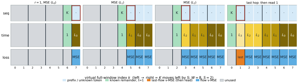
图 6: RELF clean 续写 ( W=8 , S=2 , r=1 )。虚拟满窗左切：绿格 K 第一帧在 k=6 （靠右），之后每次左移 S 。红框为即将读出的新词：全程打 v-MSE，末流档 L_{T-1} Euler 后才读出。末帧 K 在 k=0 ，即混合窗 F ，对应图 5。不画第一次 pop 之后的 freeroll。
