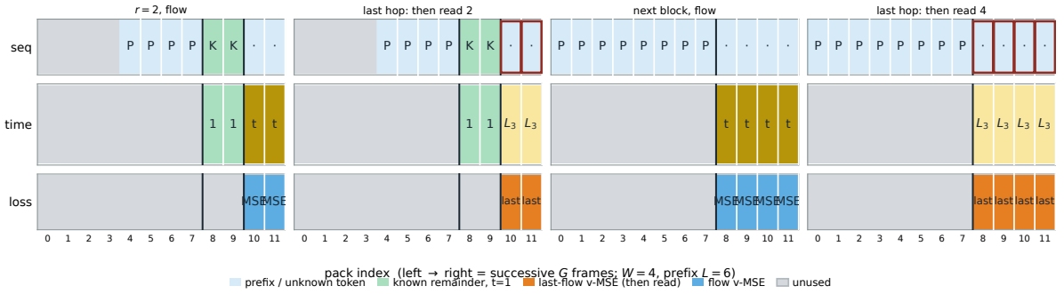
图 2: BELF clean 续写 ( W = 4 , 前缀 L = 6 故 r = 2 )。从左到右为相继的 G 帧。在混合块未知槽上走完流后读出 2 个新词；提交后下一块整块未知。绿格为块内已知余数 ( t = 1 , 不进损失)。流跳只画一帧（未知槽同一 t ）。红框为该帧读出的新词。
