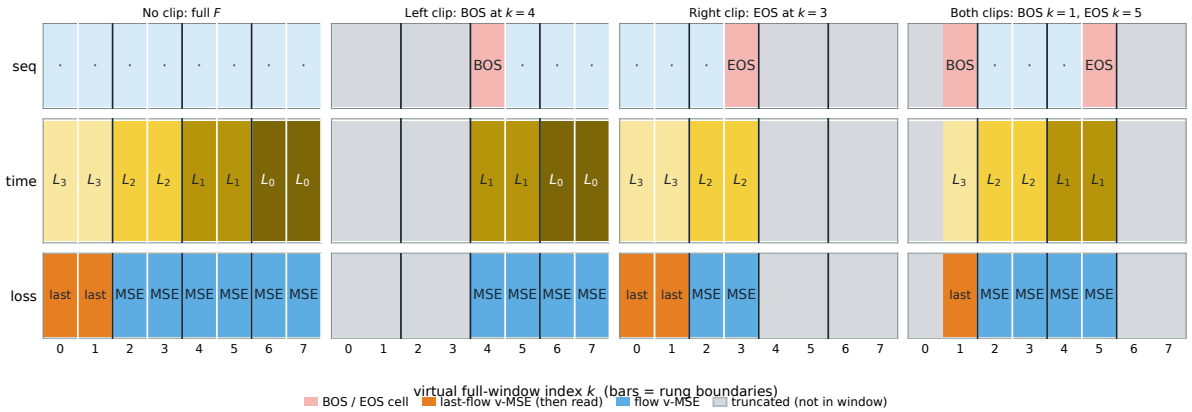
图 8: RELF 画的是虚拟满窗 F ( W = 8 , 每档 2 槽)。黄净、黑噪。橙 = 最左流档 t = L_{T-1} (该步 Euler 到 1 - \varepsilon 后读出)；蓝 = 更噪流档。灰格是 BOS 之前或 EOS 之后，不在窗、不赋 t = 0 。前三列是只切一侧或不切；右列两端都切。损失按切完后的 F_k 按格计算，不是三选一。
