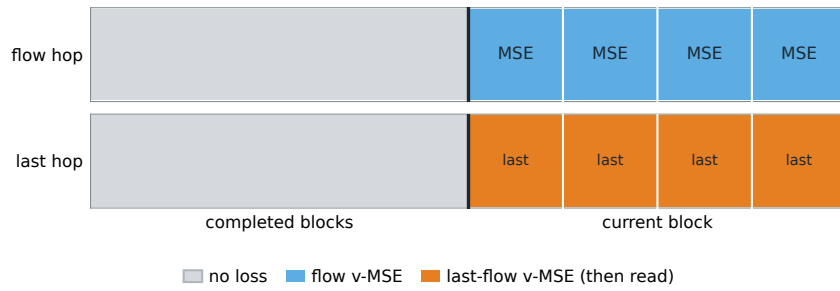
图 4: BELF: 已完成的前块不算损失。 T 次流的未知槽都算速度 MSE。橙为末流档（该步 Euler 后读出），仍是 v-MSE。
