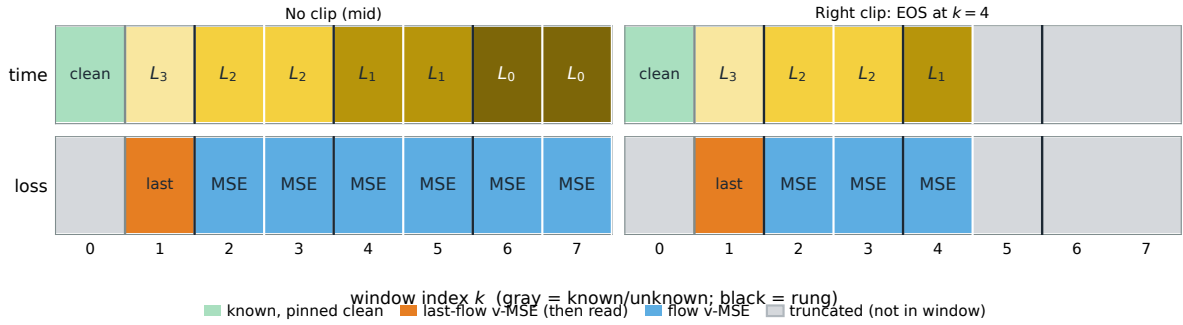
图 5: RELF clean 末帧 ( h = T - 1 ): 余数已在虚拟 k = 0 ，最左流档 Euler 后才读出。左列句中满窗；右列句尾切（EOS 后截掉， F 不滑）。这是爬梯的最后一帧，不是续写全过程。
