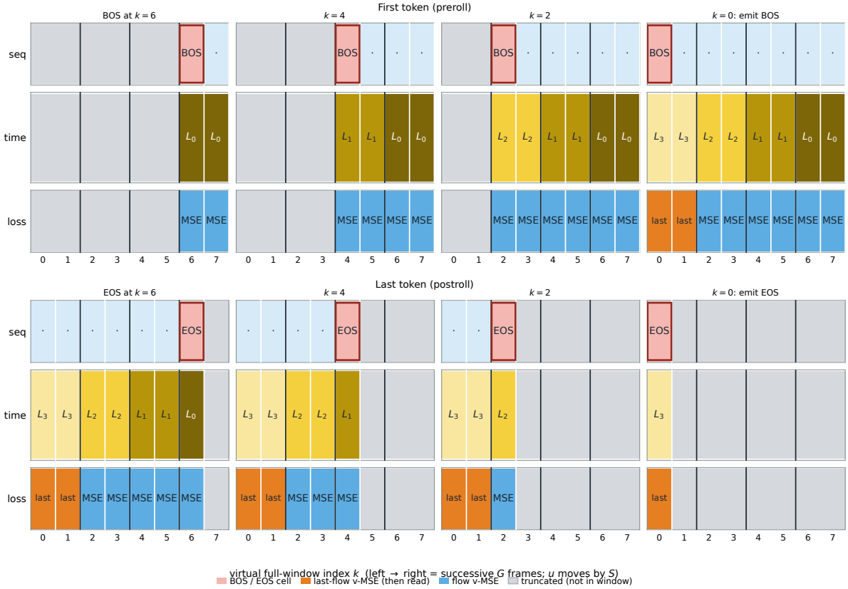
图 9: RELF 推理吐词 ( W = 8 , 每档 S = 2 )。上行句首切：窗起点 u 每次右移 S ，BOS 在虚拟满窗上左移；前三帧最左流档仍在 BOS 之前（已截掉），无读出；末帧 BOS 落到 k = 0 ，该档 Euler 后 VAE-dec 并 pop 出首词。下行句尾切：EOS 之后丢掉、不再右补噪声；EOS 左移，末帧只剩 k = 0 的 EOS，VAE-dec 读出。灰格不在窗，不赋 t = 0 。
