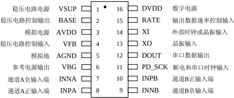
SOP-16L 封装
