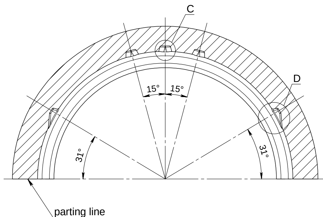
SECTION A-A
