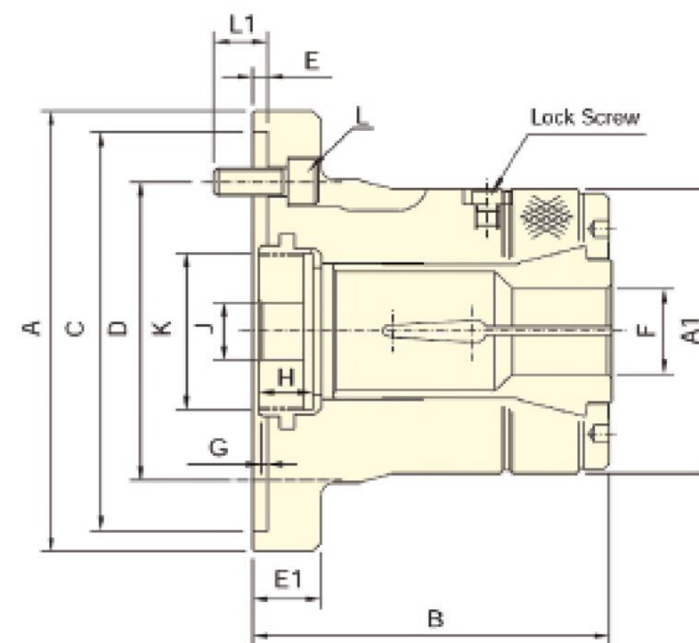
Исполнение с цилиндрической посадкой
