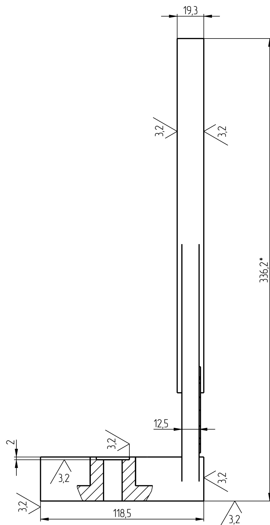
B-B
