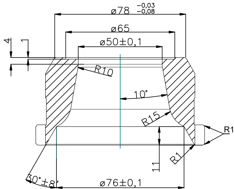
PREREZ A-A
