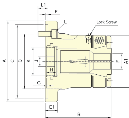
Исполнение с цилиндрической посадкой
