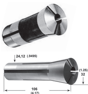
Тип 369 E (R8)
