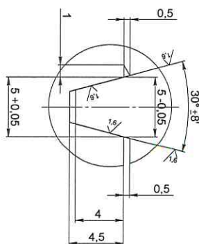
DETAIL A-A
