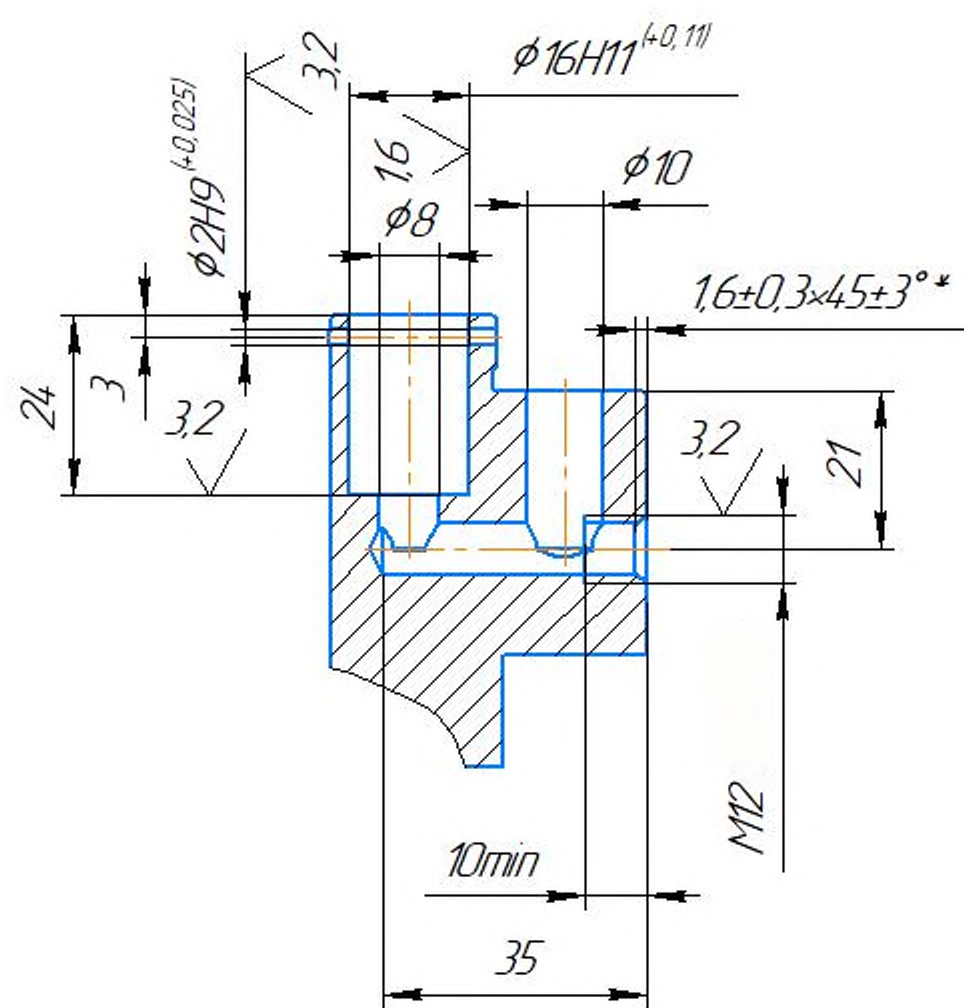
Д-Д
