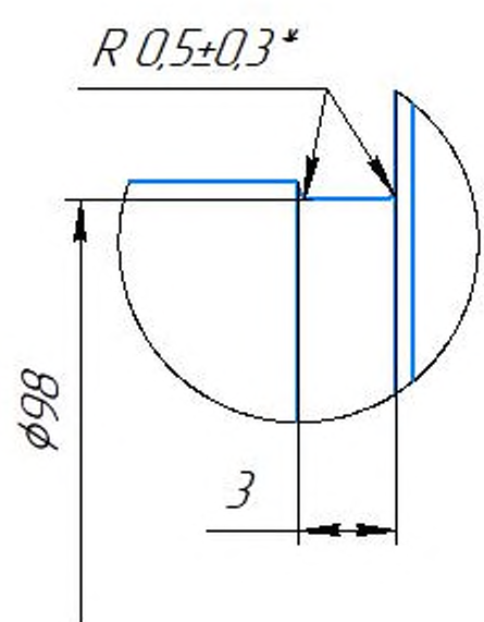
В (4:1)
