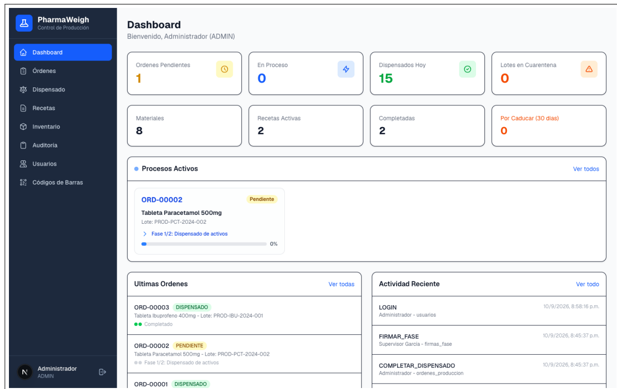
Dashboard principal: KPIs, órdenes recientes y actividad del sistema.
