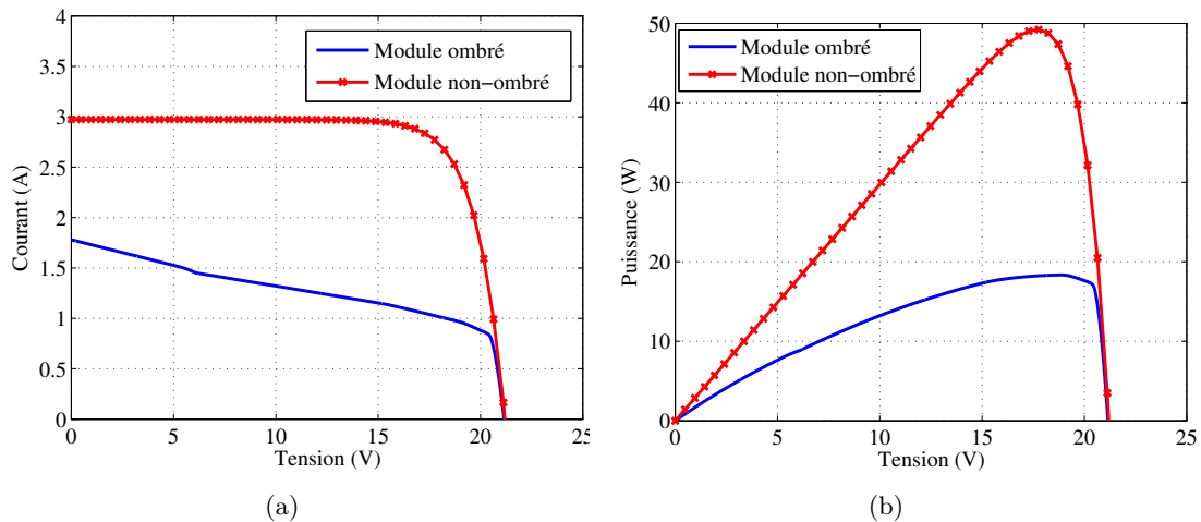
FIGURE III.17 – Comparaison entre les caractéristiques électrique d'un module ombré et non ombré.(a) les caractéristiques ( I - V ). (b) les caractéristiques ( P - V ).
