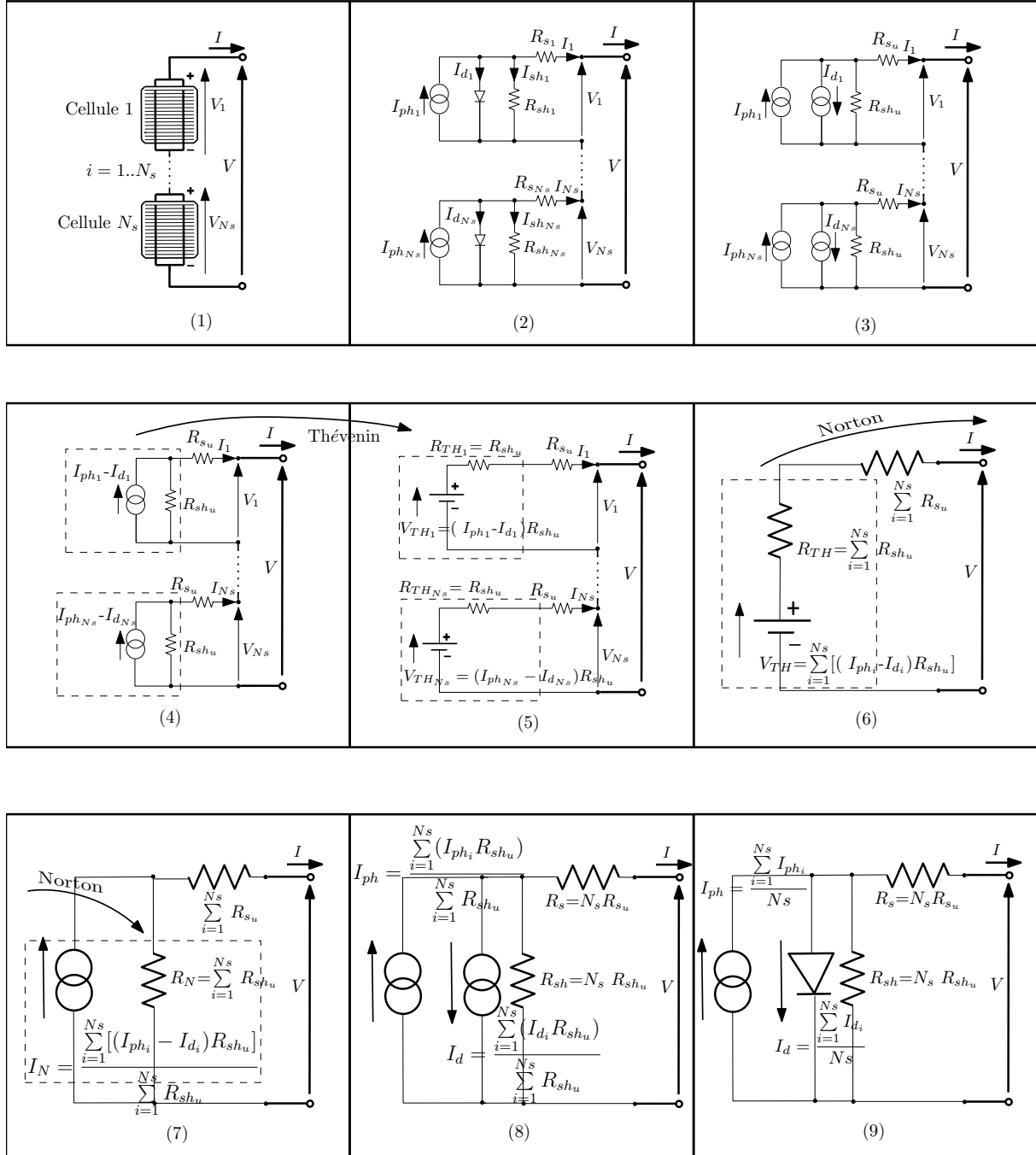
FIGURE III.4 – Illustrations avec démonstration d'une association en série de N_s cellules solaires.
