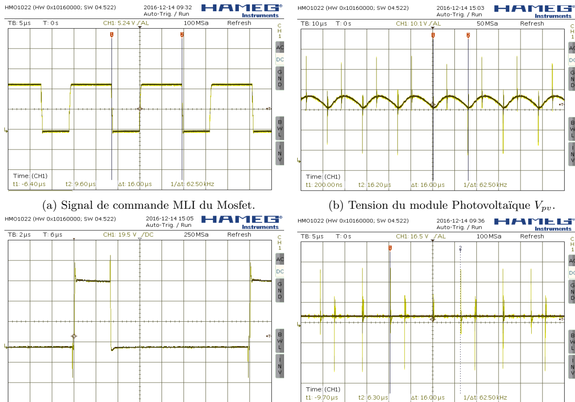
(a) Signal de commande MLI du Mosfet. (b) Tension du module Photovoltaïque V_{pv} . (c) Tension entre le Drain et la Source du Mosfet V_{ds} . (d) Tension de sortie aux bornes de la charge V_s .
