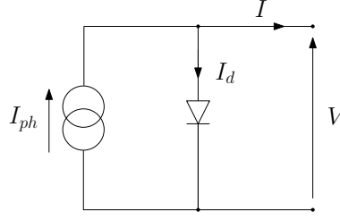
FIGURE II.5 – Circuit électrique équivalent du modèle idéal.
