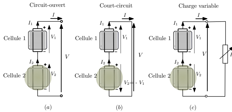
FIGURE III.9 – Illustration de l'effet de maladaptation sur deux cellules solaires connectées en série.
