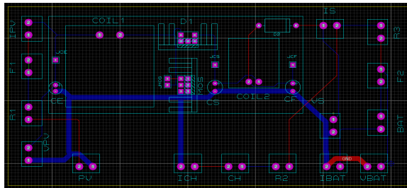
(c) Routage des pistes du circuit imprimé en utilisant Proteus ARES.
