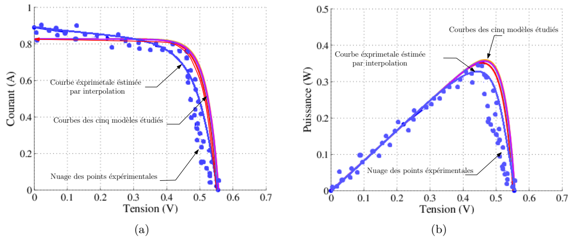
FIGURE II.22 – Comparaison entre les différents modèles et la courbe expérimentale : (a) la caractéristique ( I-V ). (b) la caractéristique ( P-V )
