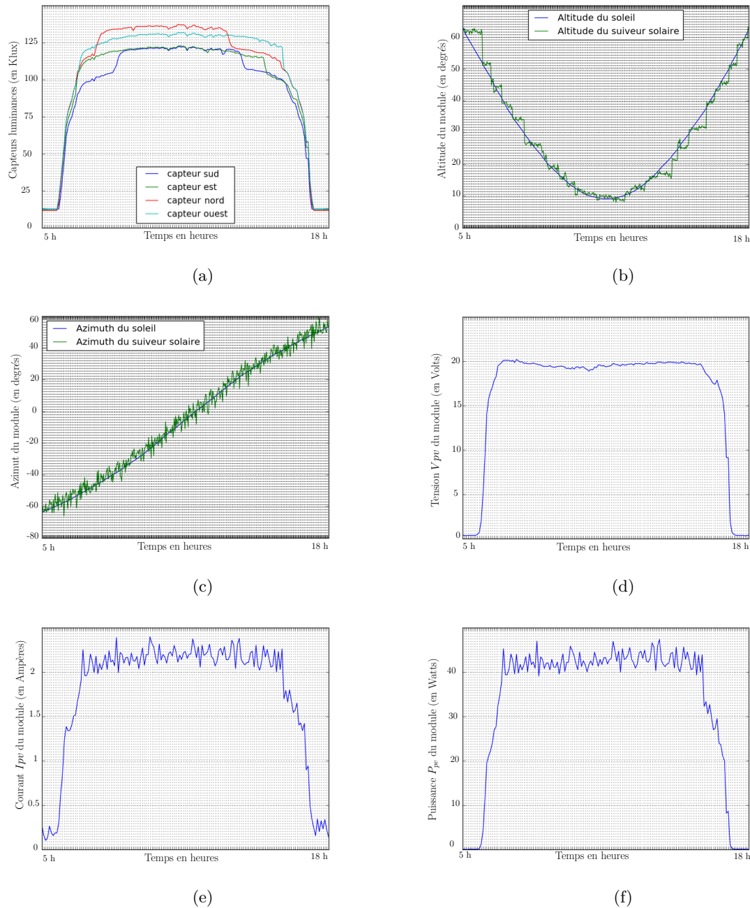
FIGURE V.5 – Résultats expérimentaux du suiveur solaire en 6 novembre 2016.
