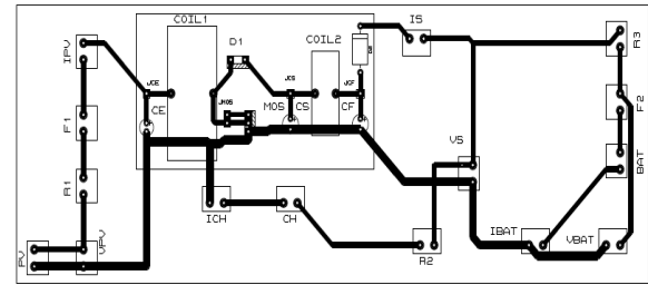
(d) Typon du circuit imprimé du régulateur de charge.
