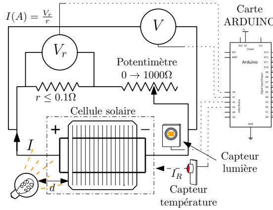
FIGURE II.3 – Schéma explicatif de la méthode de mesures de la cellule solaire “JAC M5SF-2”.
