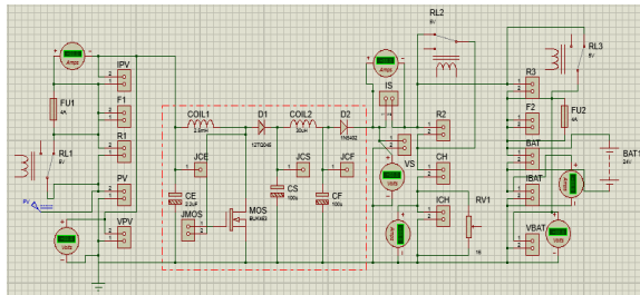
(a) Circuit schématique de la carte de puissance contenant le convertisseur Boost en utilisant Proteus ISIS .
