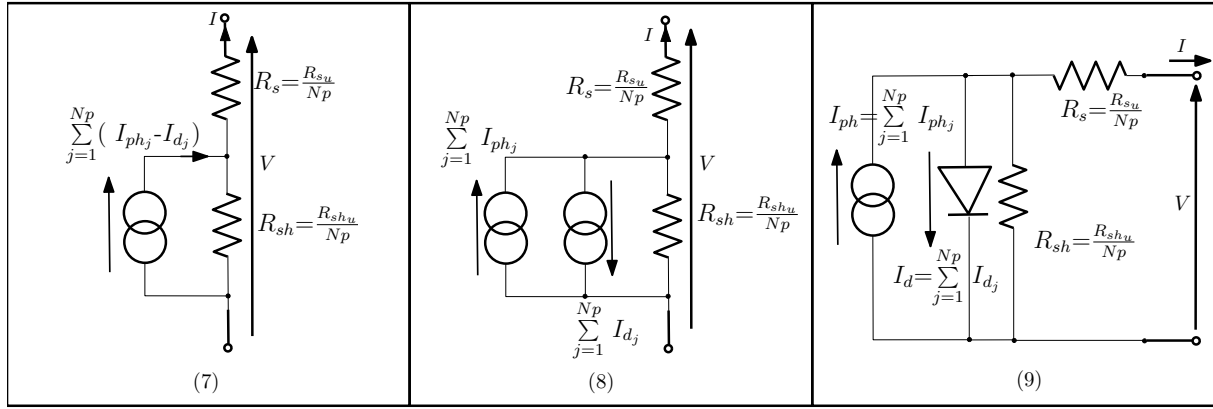
FIGURE III.5 – Illustrations avec démonstration d'une association en parallèle de N_p cellules solaires.
