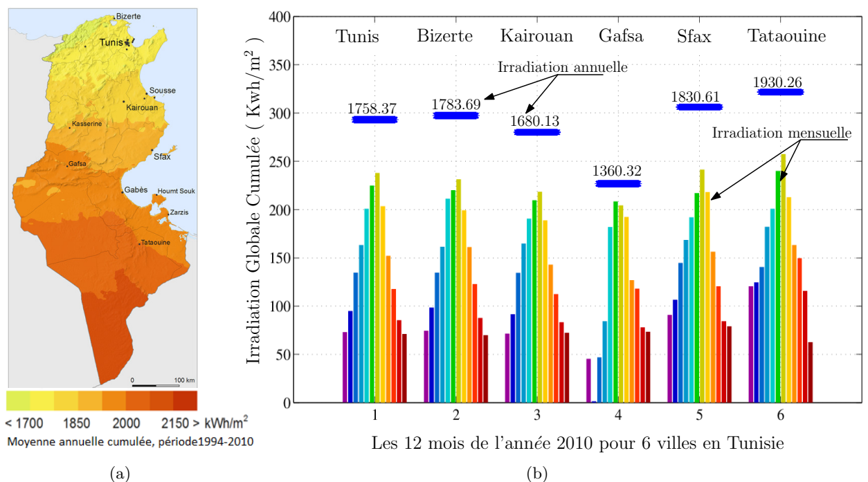
FIGURE III.19 – Gisement Solaire en Tunisie. (a) Irradiation Globale Horizontale en KWh/m 2 en Tunisie (Source : Solargiz). (b) Irradiation Globale cumulée par mois et par année en KWh/m 2 en six villes de la Tunisie (Source : INM).
