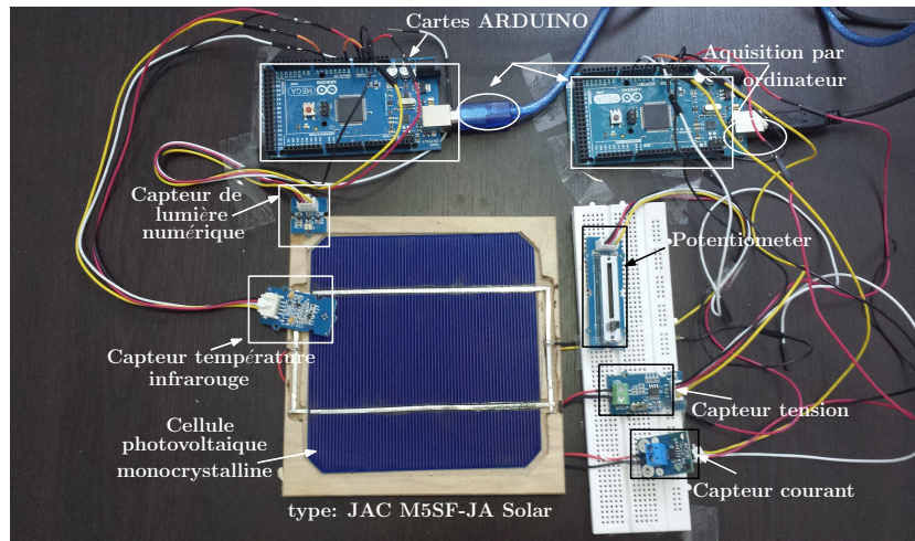
FIGURE II.4 – Banc d'essai expérimental de la cellule solaire “JAC M5SF”.
