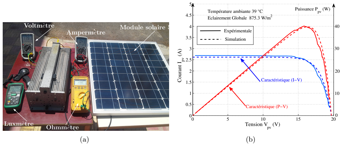
FIGURE III.7 – Module solaire 50W utilisé.(a) Banc d'essai des tests expérimentaux.(b) Comparaisons entre les caractéristiques électriques expérimentales et de simulations
