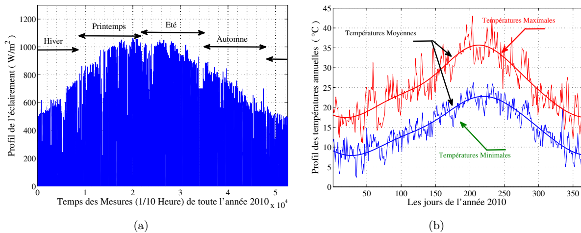
FIGURE III.20 – Caractéristiques Solaire de la ville de Sfax. (a) Profil du rayonnement solaire de l'année 2010 en W/m^2 . (b) Profil de la fourchette des températures de l'année 2010. (Source : INM).
