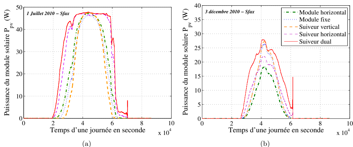
FIGURE III.27 – Simulation des suiveurs solaires durant la meilleure et la pire journées d’éclairement en 2010 à Sfax. (a) Puissances générées pendant la meilleure journée. (b) Puissances générées pendant la pire journée.
