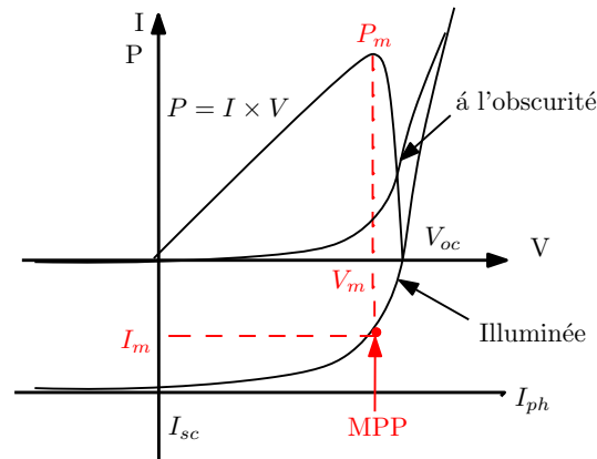
FIGURE I.7 – Caractéristique d'une cellule solaire à l'obscurité et sous éclaircissement.
