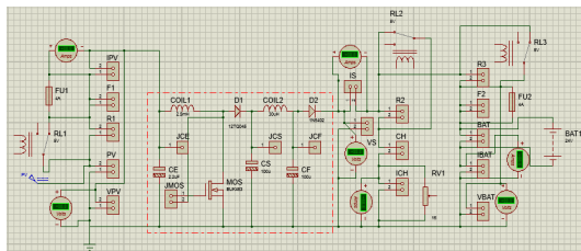
(a) Circuit schématic par Proteus ISIS de la carte de puissance contenant le convertisseur Boost .
