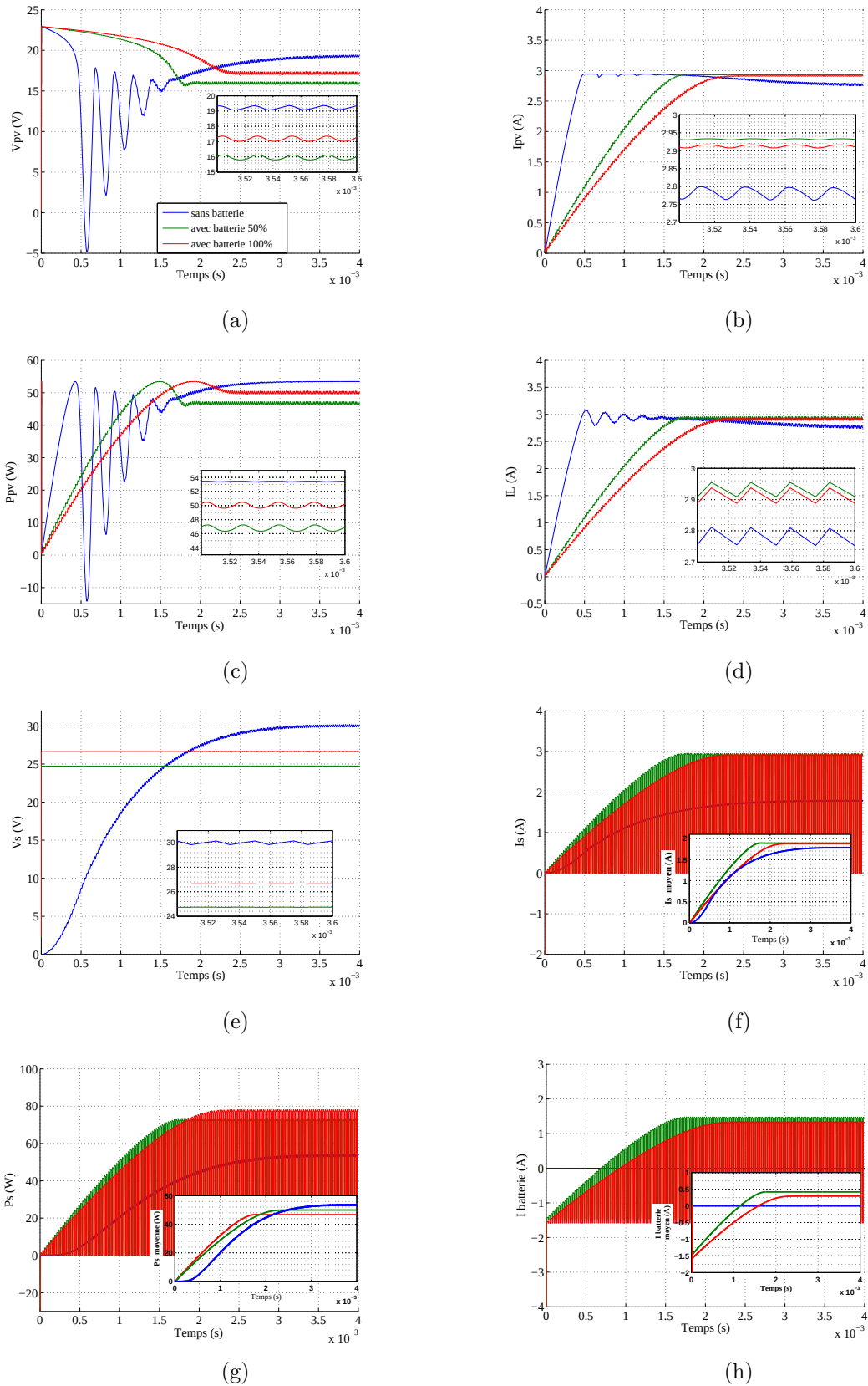
Figure IV.16: Résultats de simulation du convertisseur boost avec des composants idéaux. (a) Tension du module PV V_{pv} . (b) Courant du module PV I_{pv} . (c) Puissance du module PV P_{pv} . (d) Courant dans l'inductance I_L . (e) Tension de sortie V_S . (f) Courant de sortie I_S . (g) Puissance de sortie P_S . (h) Courant de la batterie I_{bat} .
