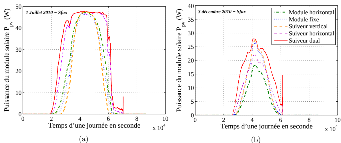
Figure III.27: Simulation des suiveurs solaires durant la meilleure et la pire journées d'éclairage en 2010 à Sfax. (a) Puissances générées pendant la meilleure journée. (b) Puissances générées pendant la pire journée.
