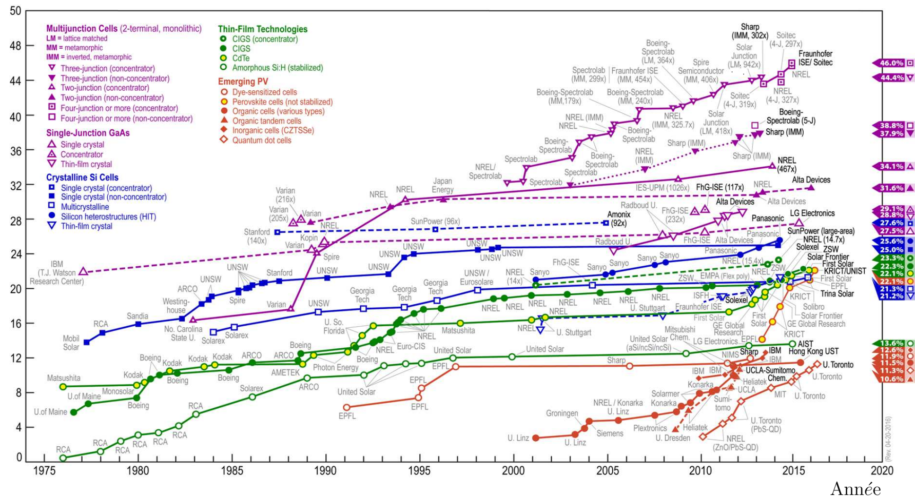
Figure I.2: Développement des records des rendements des cellules solaires au cours des 40 dernières années (source : NREL).
