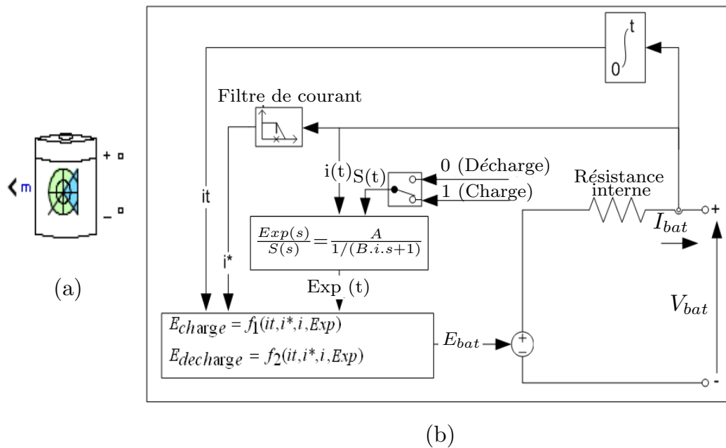
Figure IV.6: Modèle électrique de batterie de la boîte à outil SimPowerSystems . (a) Symbolisation. (b) Schéma électrique.
