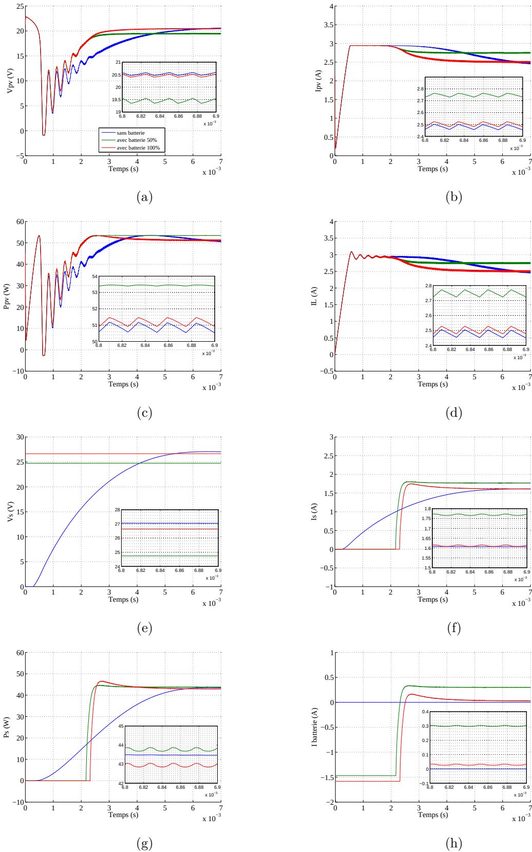
Figure IV.18: Résultats de simulations du convertisseur boost en tenant compte des pertes de puissance.
