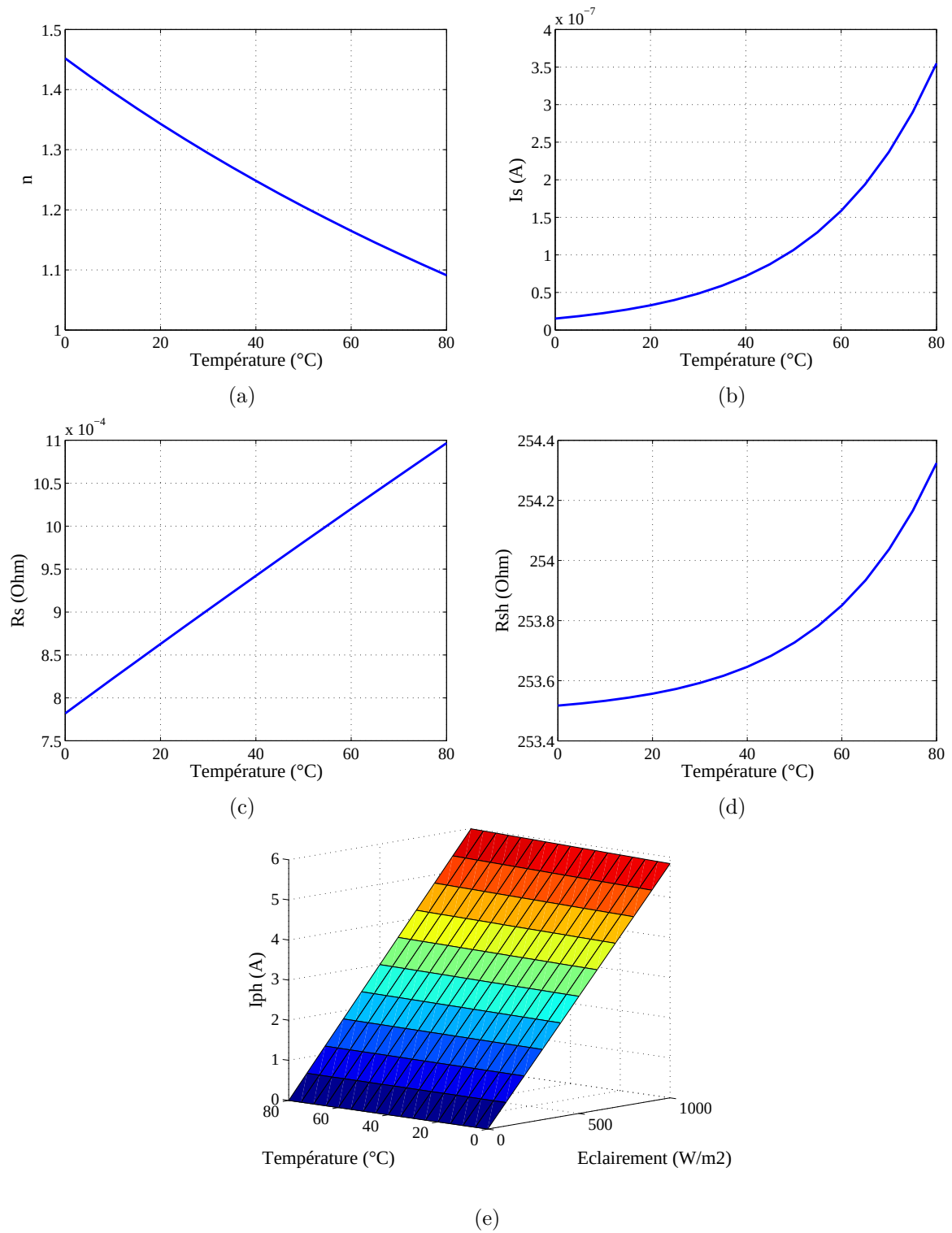
Figure II.12: Variations des paramètres internes du modèle à une diode de la cellule solaire JAC M5SF-2 en fonction de la température et de l'éclairement. (a) Variations de n en fonction de la température. (b) Variations de I_s en fonction de la température. (c) Variations de R_s en fonction de la température. (d) Variations de R_{sh} en fonction de la température. (e) Variations de I_{ph} en fonction de la température et de l'éclairement.
