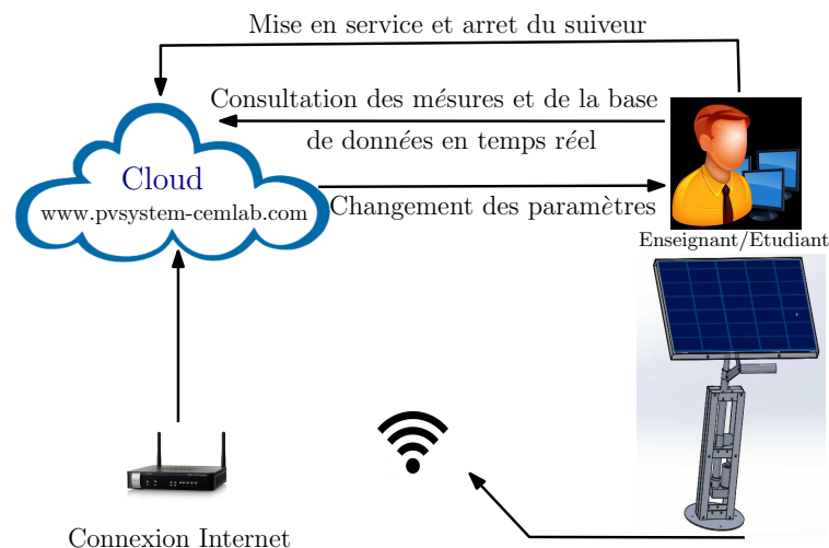
Figure V.2: Processus d'acquisition des données.
