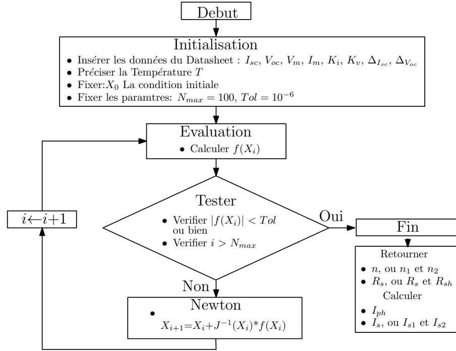
Figure II.9: Algorithme de recherche des paramètres internes des modèles : à une résistance série, à une diode et à deux diodes.
