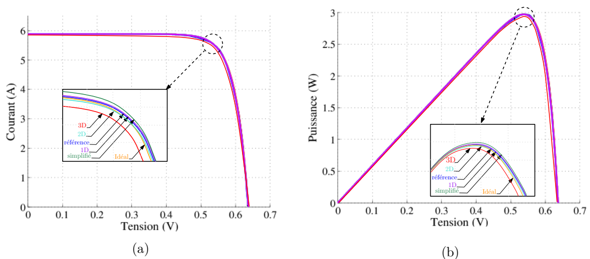
Figure II.21: Comparaison entre les différents modèles et la courbe de référence : (a) la caractéristique (I-V). (b) la caractéristique (P-V)
