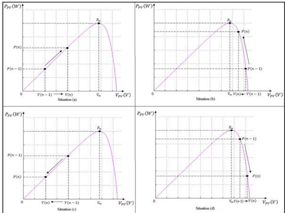
Figure IV.19: Différentes situations considérées par la stratégie MPPT.
