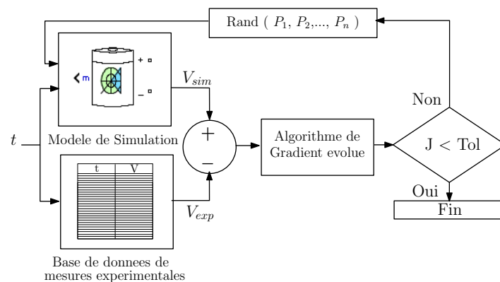
Figure IV.9: Schéma explicatif de la méthode d'ajustement des courbes utilisée pour l'identification des paramètres de la batterie “Power Kingdom PS7-12”.
