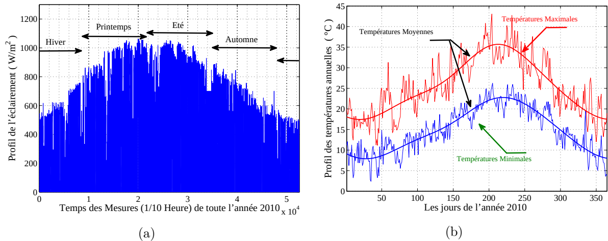
Figure III.20: Caractéristiques Solaire de la ville de Sfax. (a) Profil du rayonnement solaire de l'année 2010 en \text{W/m}^2 . (b) Profil de la fourchette des températures de l'année 2010. (Source : INM).
