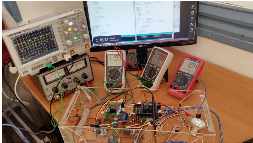
Figure V.9: Test du système de régulation de charge.
