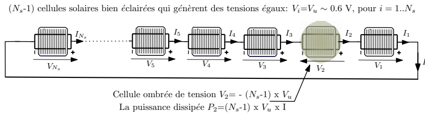
Figure III.11: Illustrations du phénomène du “Hot-spot”
