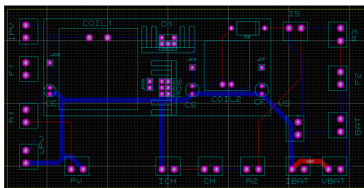
(a) Routage des piste du circuit imprimé en utilisant Proteus ARES.
