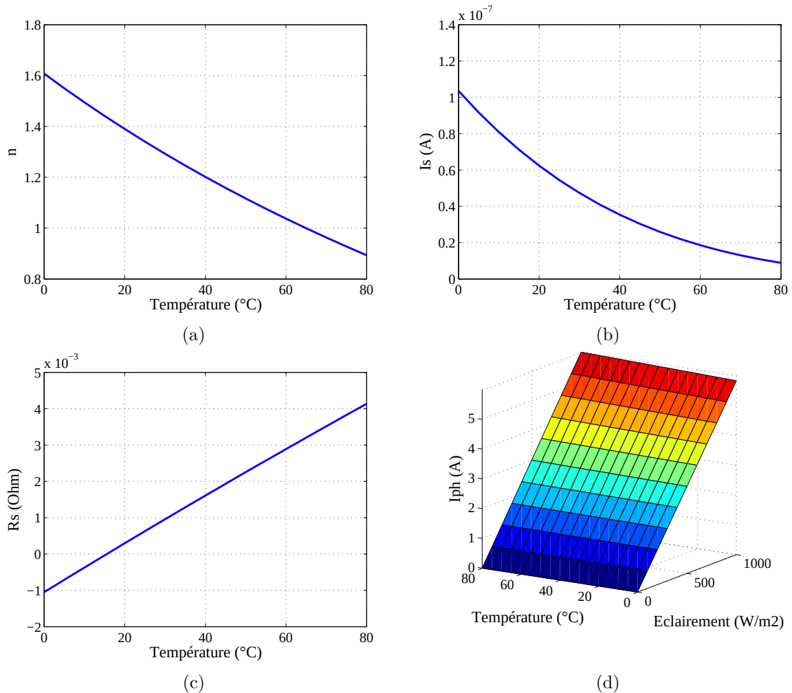
Figure II.10: Variations des paramètres internes du modèle à une résistance série de la cellule solaire JAC M5SF-2 en fonction de la température et de l'éclairement. (a) Variations de n en fonction de la température. (b) Variations de I_s en fonction de la température. (c) Variations de R_s en fonction de la température. (d) Variations de I_{ph} en fonction de la température et de l'éclairement.
