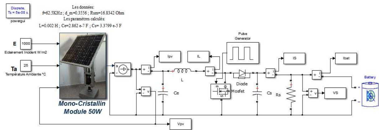
Figure IV.15: Modèle de simulation de la Chaîne PV à travers des composants idéaux.
