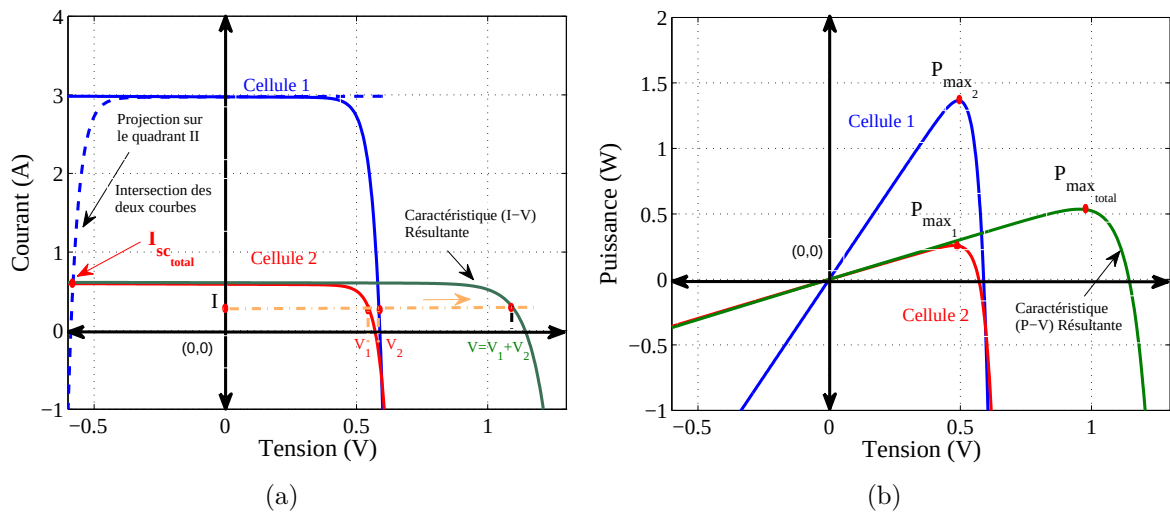
Figure III.10: Caractéristiques électriques de maladaptation sur deux cellules solaires connectées en série. (a) Caractéristiques (I - V) . (b) Caractéristiques (P - V) .
