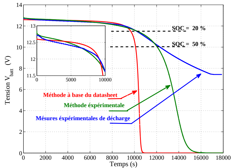
Figure IV.10: Comparaison les caractéristiques de décharge de la batterie "Power Kingdom PS7-12".
