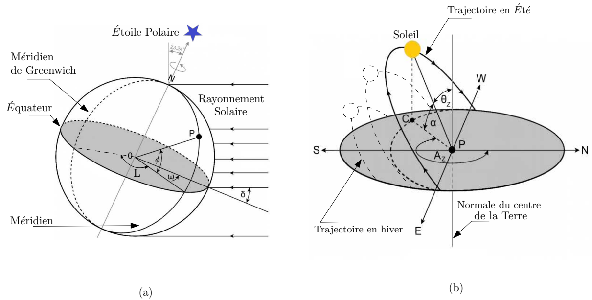
Figure III.21: Mouvement apparent du soleil. (a) Les angles d'un point P de la Terre. (b) Les angles du soleil vue par le point P . (Source : ITACA) 3
