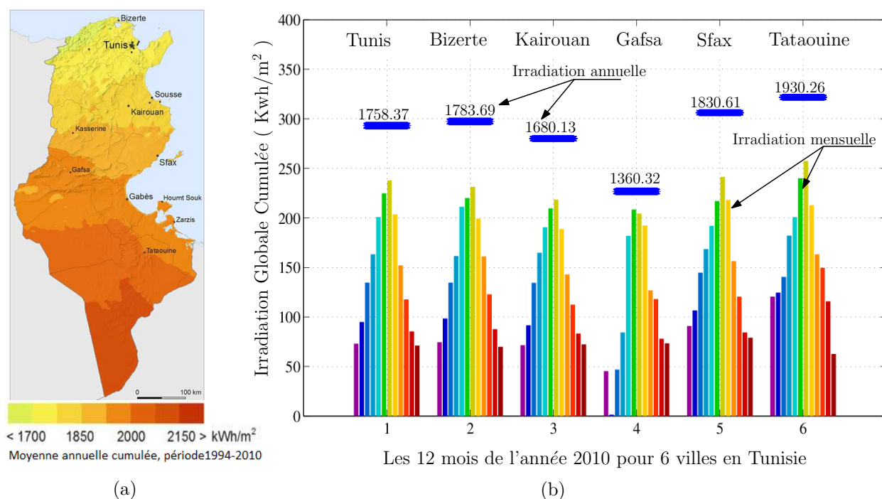
Figure III.19: Gisement Solaire en Tunisie. (a) Irradiation Globale Horizontale en KWh/m 2 en Tunisie (Source : Solargiz). (b) Irradiation Globale cumulée par mois et par année en KWh/m 2 en six villes de la Tunisie (Source : INM).
