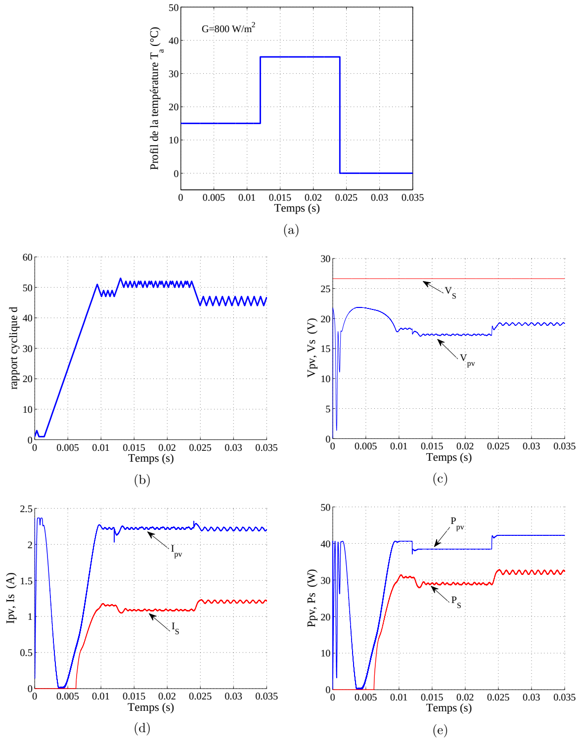
Figure IV.24: Effet de la variation de la température sur les grandeurs électriques de la chaîne de conversion PV. (a) Profil de température. (b) Rapport cyclique. (c) Tensions d'entrée V_{pv} et de sortie V_s . (d) Courants d'entrée I_{pv} et de sortie I_s . (e) Puissances d'entrée P_{pv} et de sortie P_s
