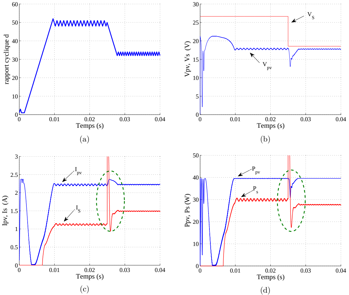
Figure IV.22: Effet de la variation de la charge sur les grandeurs électriques de la chaîne de conversion PV. (a) Rapport cyclique. (b) Tensions d'entrée V_{pv} et de sortie V_s . (c) Courants d'entrée I_{pv} et de sortie I_s . (d) Puissances d'entrée P_{pv} et de sortie P_s .
