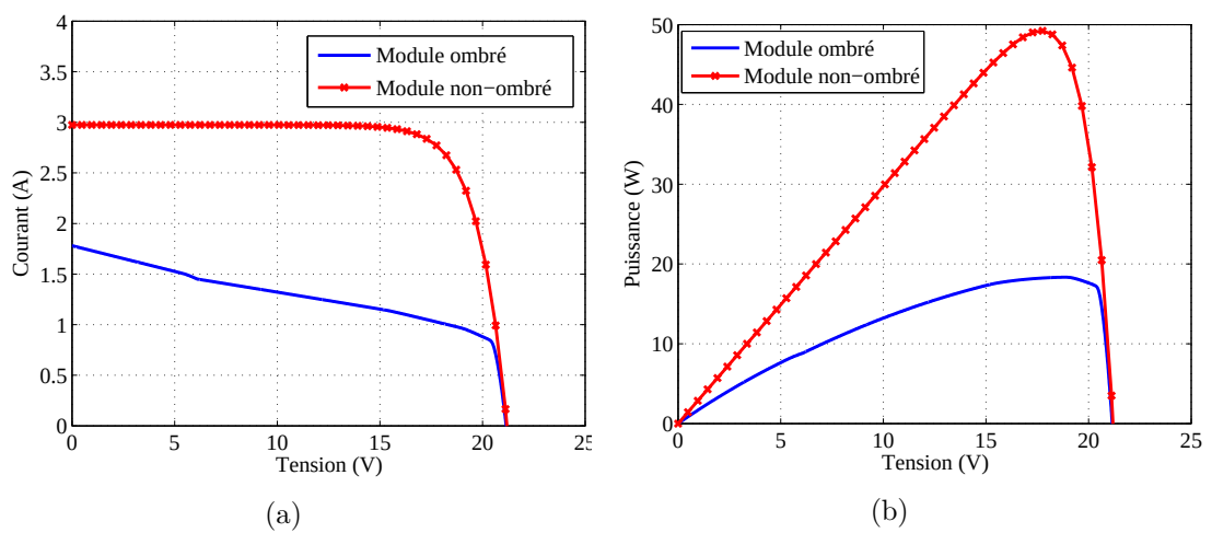
Figure III.17: Comparaison entre les caractéristiques électrique d'un module ombré et non ombré.(a) les caractéristiques ( I - V ). (b) les caractéristiques ( P - V ).
