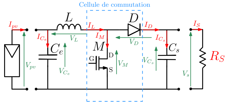
Figure IV.13: Structure du convertisseur boost.
