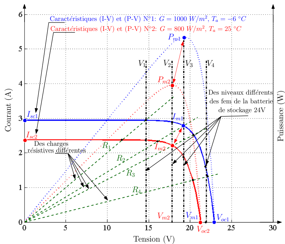
Figure IV.1: Intersections entre les niveaux des fem d'une batterie 24 V et diverses charges résistives avec les caractéristiques ( I - V ) et ( P - V ) d'un générateur PV : points de fonctionnements lors d'un couplage direct.
