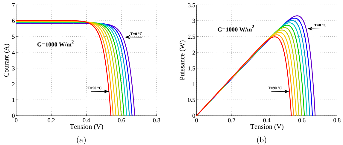
Figure II.24: Effect de la variation de la température sur les caractéristiques de la cellule solaire : (a) la caractéristique (I-V). (b) la caractéristique (P-V)
