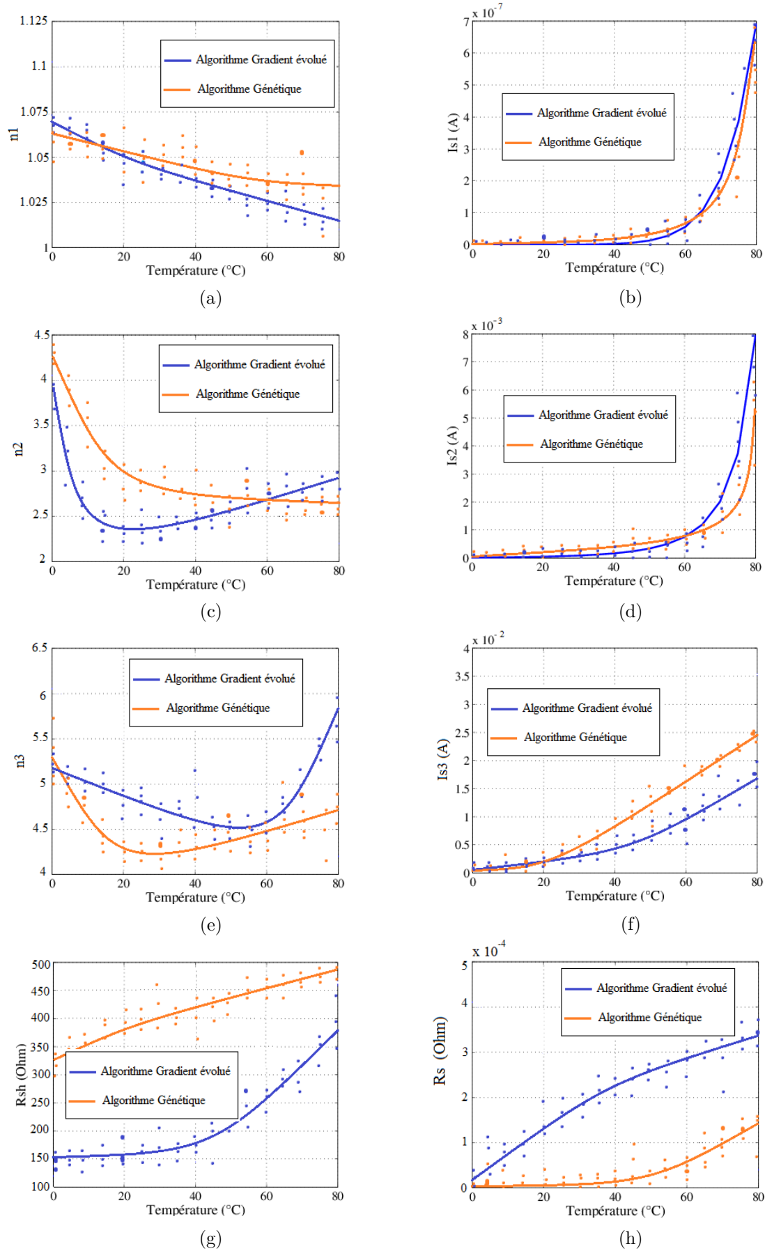
Figure II.19: Variations des paramètres internes du modèle à trois diodes de la cellule solaire JAC M5SF-2 en fonction de la température. (a) Variations de n_1 en fonction de la température. (b) Variations de I_{s1} en fonction de la température. (c) Variations de n_2 en fonction de la température. (d) Variations de I_{s2} en fonction de la température. (e) Variations de n_3 en fonction de la température. (f) Variations de I_{s3} en fonction de la température. (g) Variations de R_{sh} en fonction de la température. (h) Variations de R_s en fonction de la température.
