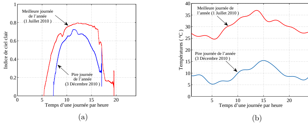
Figure III.25: Caractéristiques météorologiques durant la meilleure et la pire journées d'éclairement en 2010 à Sfax. (a) Profil de l'indice du ciel clair. (b) Profil de température réelle mesurée (°C) (Source : INM).
