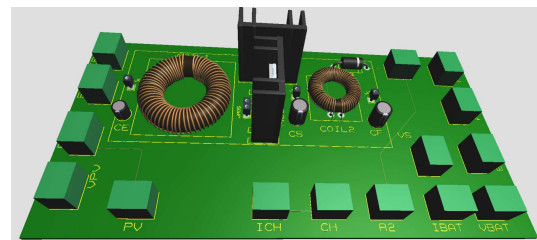
(b) Conception en 3D de la carte imprimée du convertisseur Boost.
