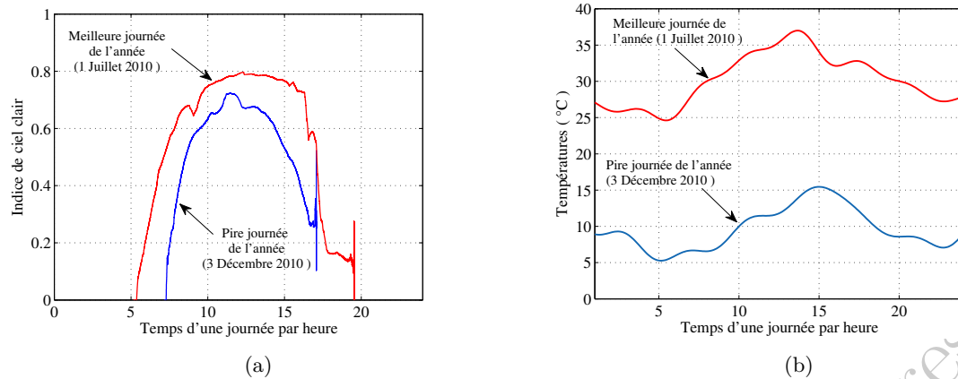
FIGURE III.25 – Caractéristiques météorologiques durant la meilleure et la pire journées d'éclairement en 2010 à Sfax. (a) Profil de l'indice du ciel clair. (b) Profil de température réelle mesurée (°C) (Source : INM).
