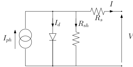
FIGURE II.11 – Circuit électrique équivalent du modèle à une diode.
