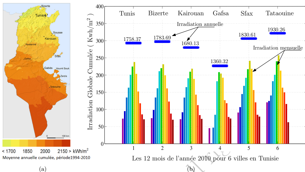
FIGURE III.19 – Gisement Solaire en Tunisie. (a) Irradiation Globale Horizontale en KWh/m 2 en Tunisie (source : Solargiz). (b) Irradiation Globale cumulée par mois et par année en KWh/m 2 dans six villes de la Tunisie (source : INM).
