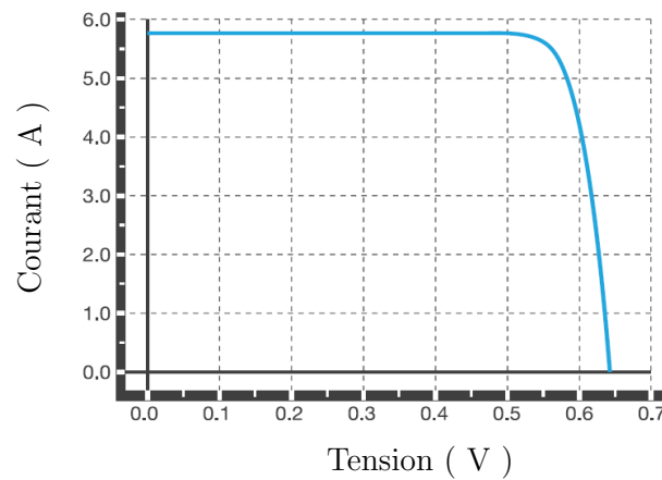
FIGURE I.8 – Caractéristique électrique ( I - V ) du fabricant de la cellule solaire “JAC M5SF-2” dans l’STC.
