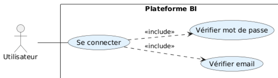
FIGURE 4.2 – Diagramme de cas d'utilisation "authentification"
