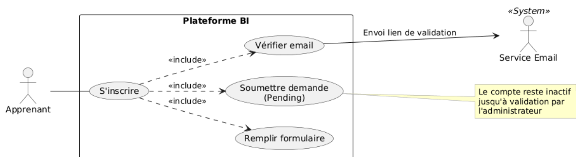
FIGURE 4.1 – Diagramme de cas d'utilisation "inscription"
