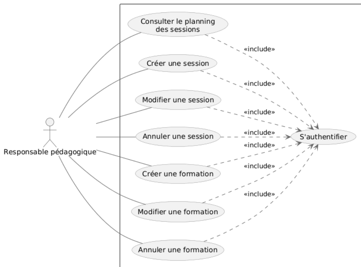
FIGURE 5.3 – Diagramme de cas d'utilisation « planning »
