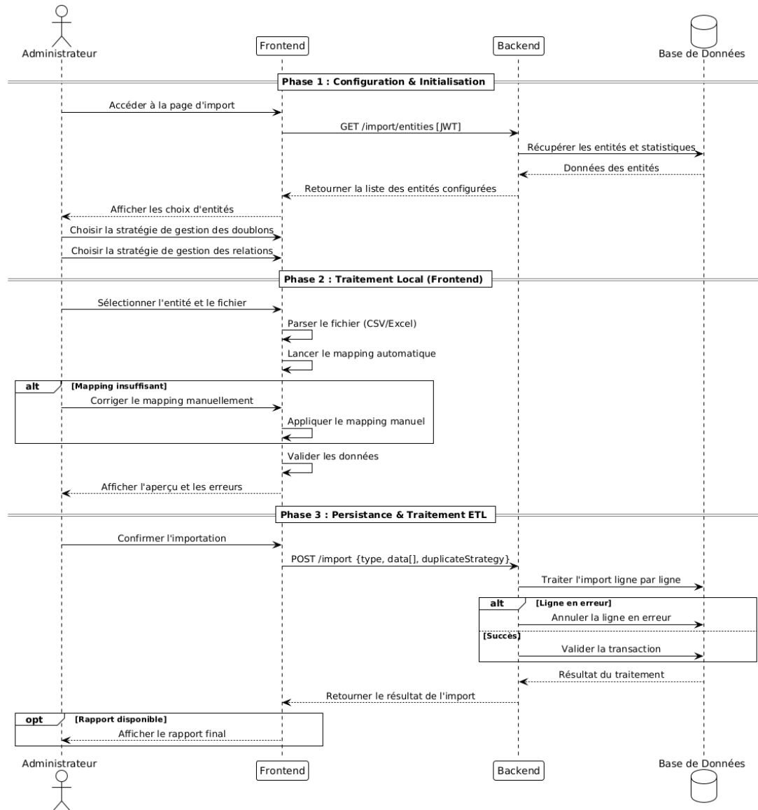
FIGURE 5.25 – Diagramme de séquence « Importer des données »
