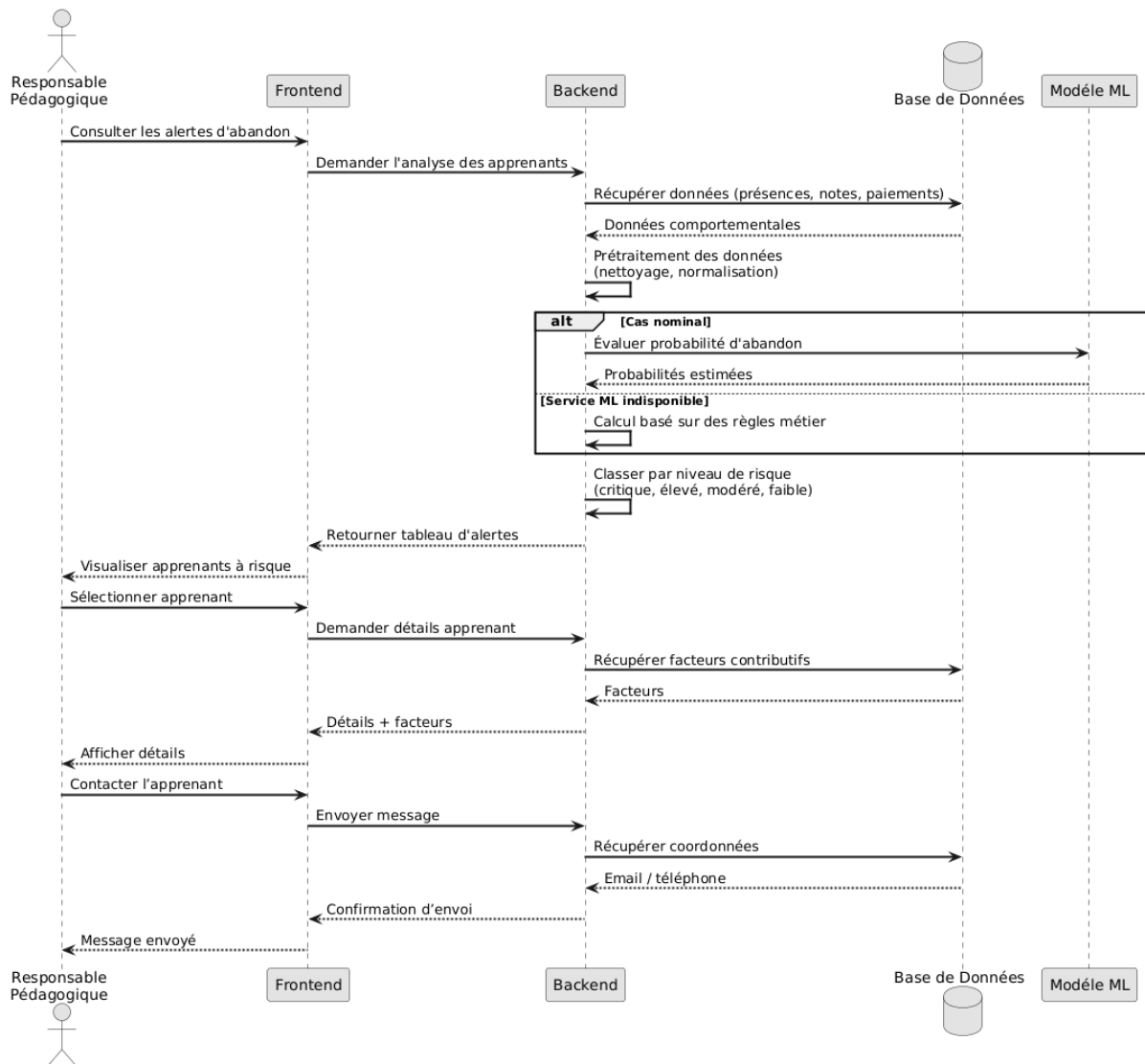
FIGURE 6.11 – Diagramme de séquence « Génération des alertes d'abandon »
