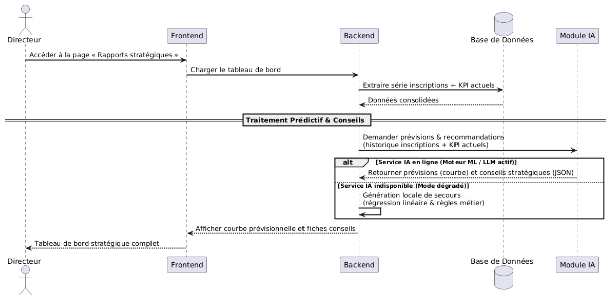
FIGURE 6.14 – Diagramme de séquence « Rapports stratégiques »
