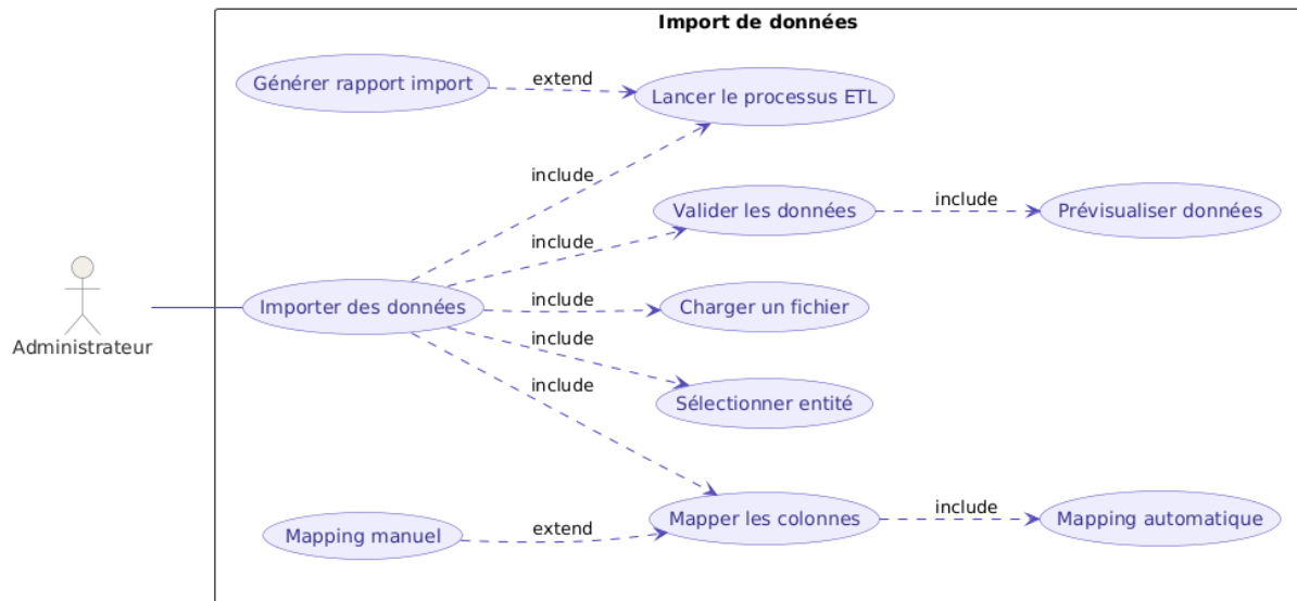
FIGURE 5.24 – Diagramme de cas d'utilisation « Importer des données »
