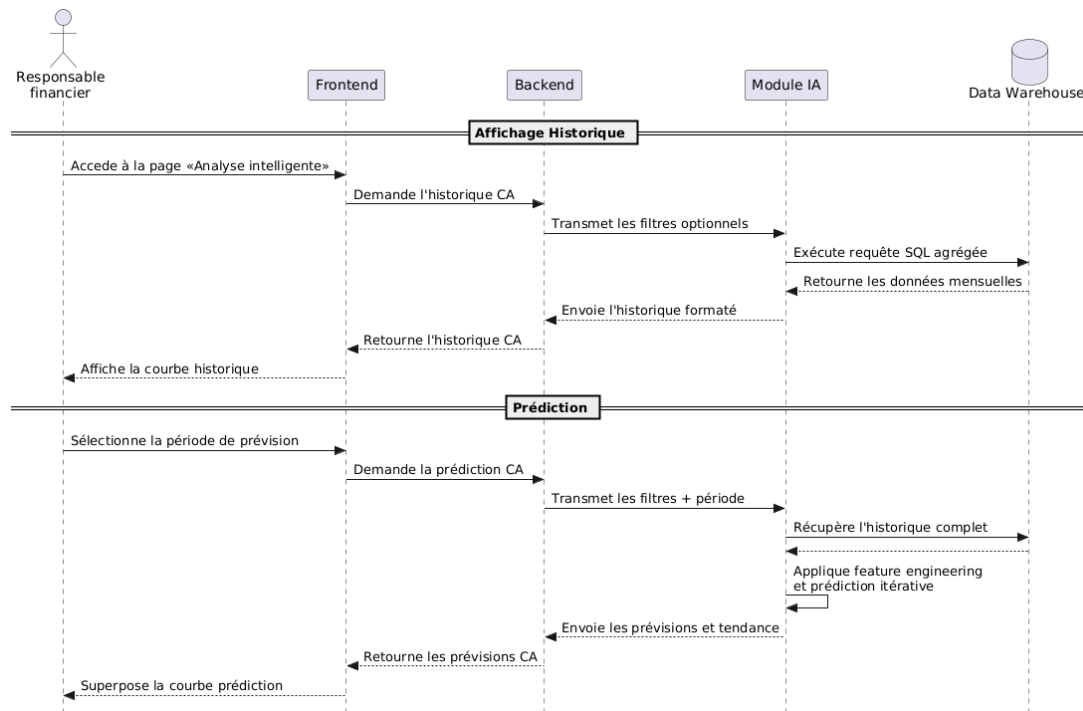
FIGURE 6.12 – Diagramme de séquence « Prédiction des revenus »
