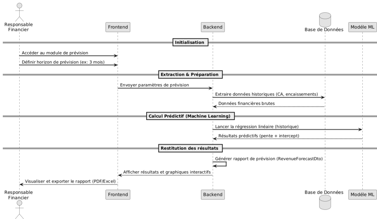
FIGURE 6.6 – Diagramme de séquence « Prédiction des revenus »
