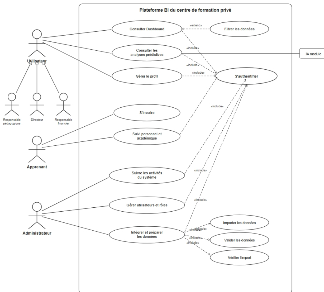
FIGURE 2.1 – Diagramme de cas d'utilisation globale
