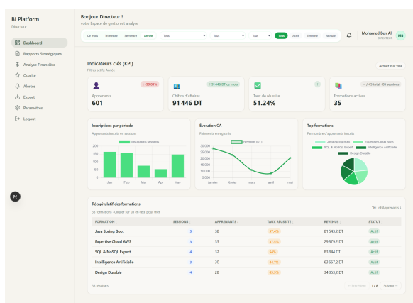
(a) tableau de bord des KPIs
