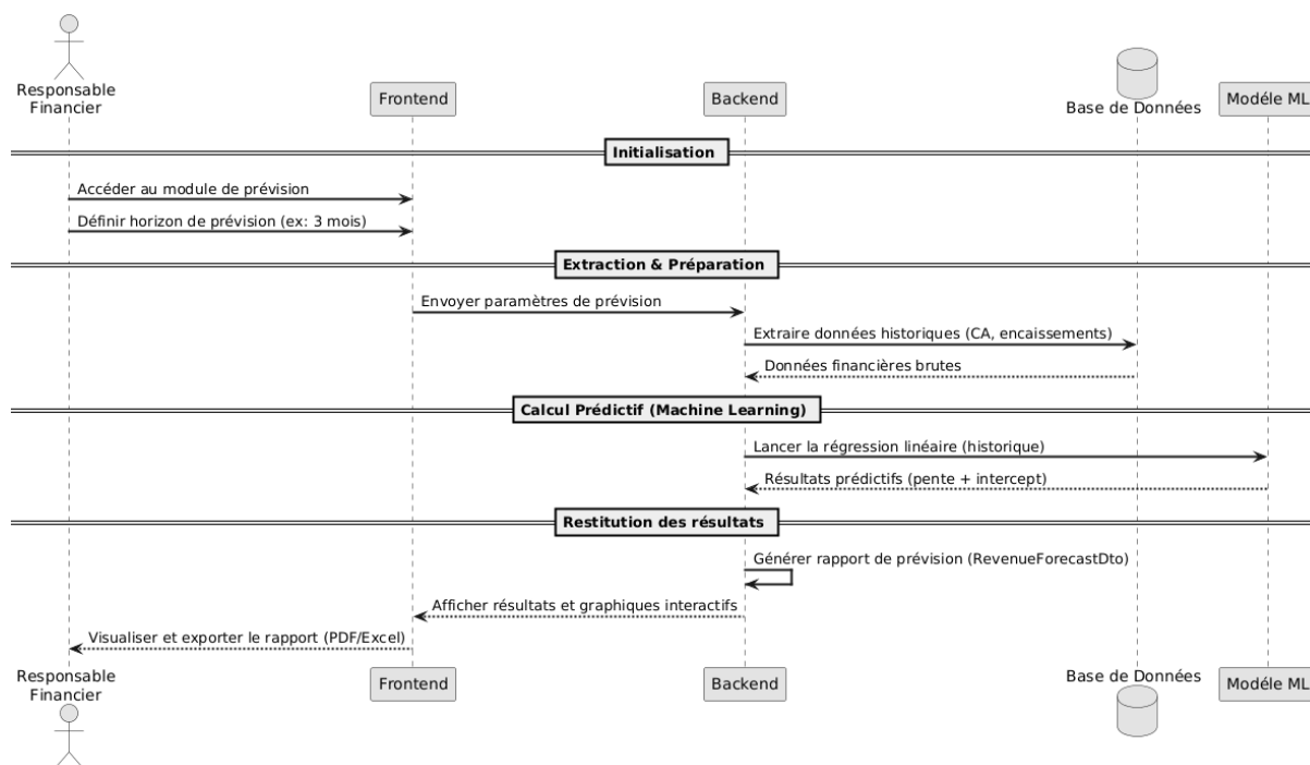
FIGURE 6.6 – Diagramme de séquence « Prédiction des revenus »
