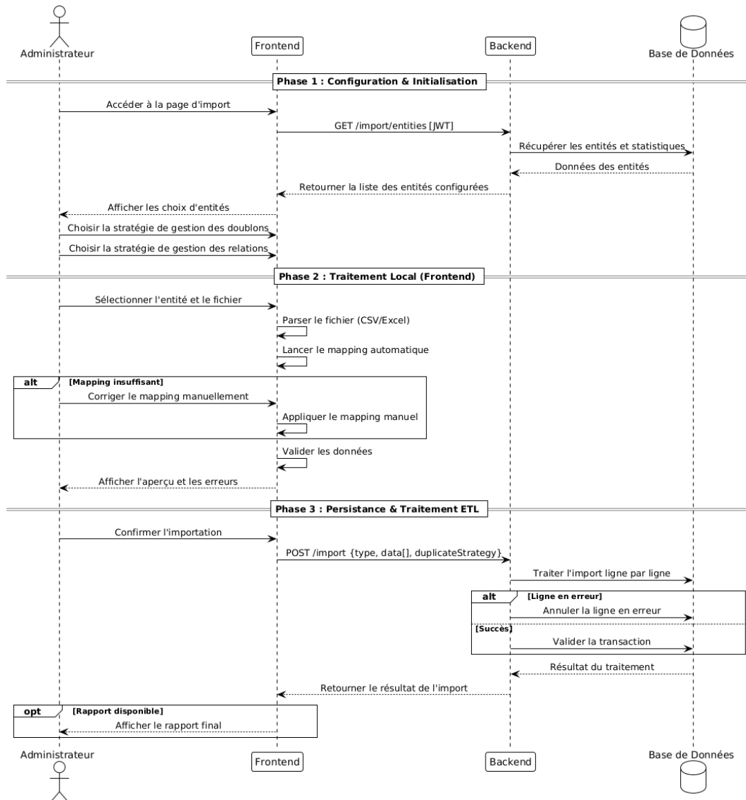
FIGURE 5.14 – Diagramme de séquence « Importer des données »
