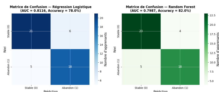
FIGURE 6.13 – Matrices de confusion — Prédiction du risque d'abandon
