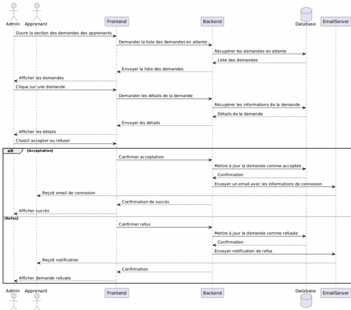
FIGURE 4.33 – Diagramme de séquence «Gestion des demandes des apprenants»
