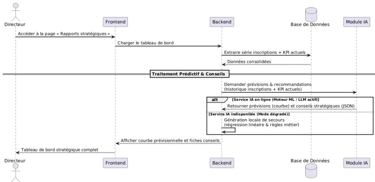
FIGURE 6.11 – Diagramme de séquence « Rapports stratégiques »
