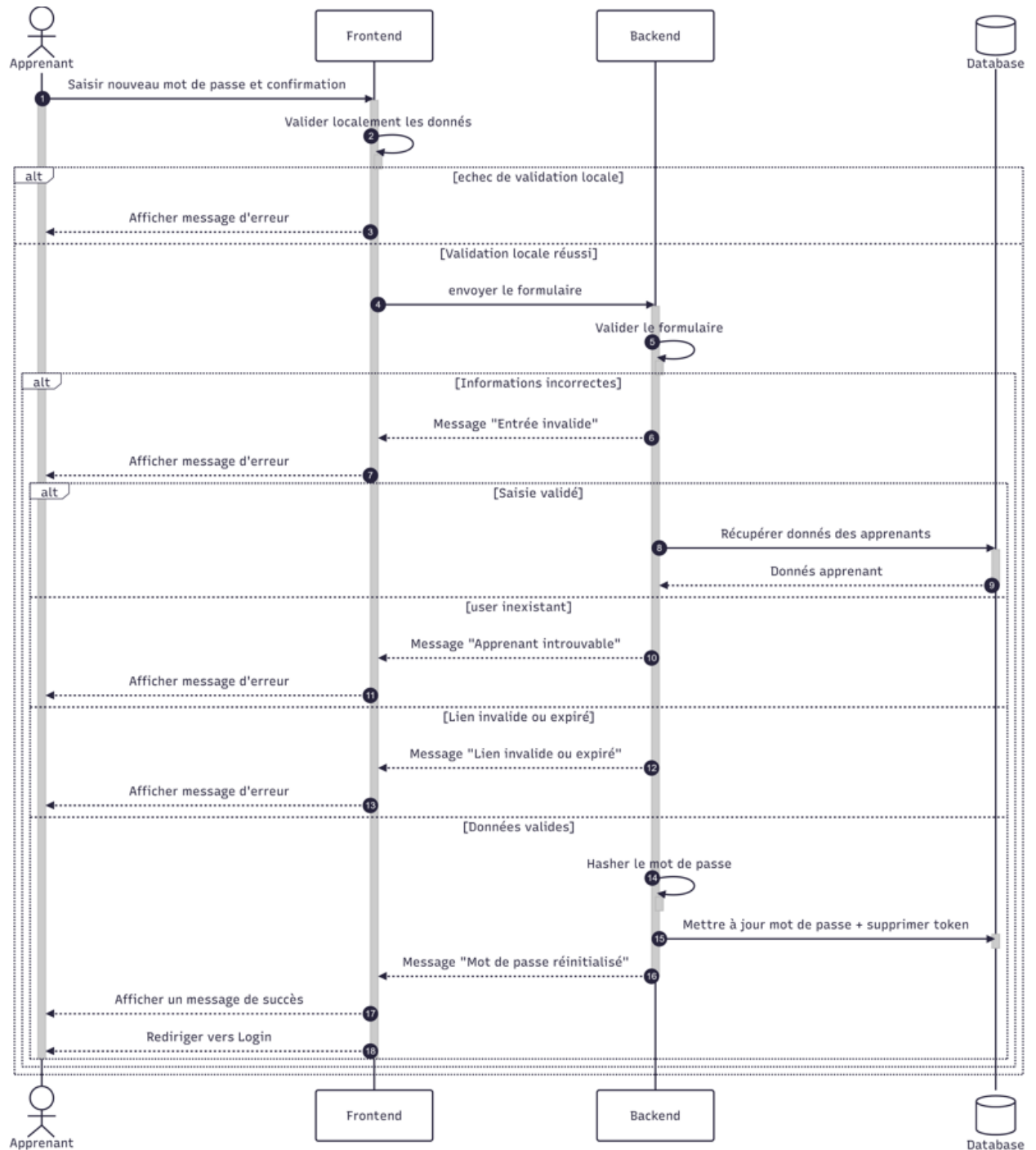
FIGURE 4.9 – Diagramme de s  quence «R  initialisation du mot de passe»
