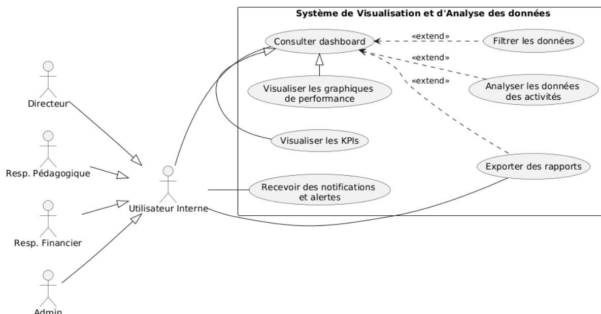
FIGURE 6.1 – Diagramme de cas d'utilisation « Visualisation et analyse des données »
