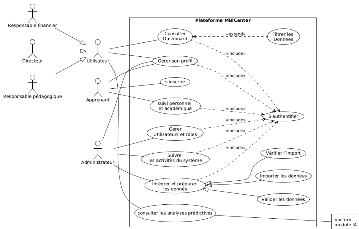
FIGURE 2.1 – Diagramme de cas d'utilisation globale
