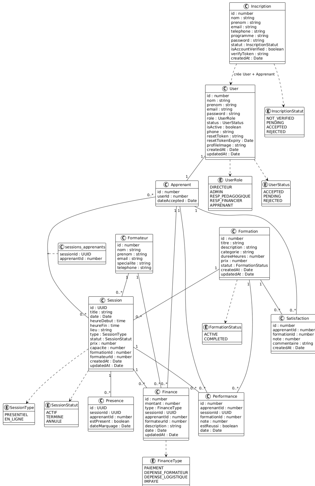
FIGURE 3.16 – Diagramme de classe
