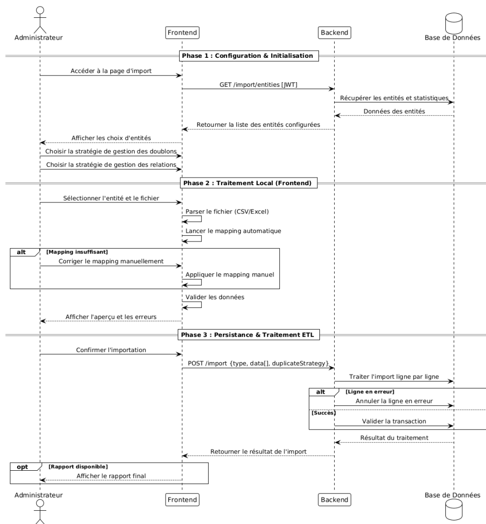
FIGURE 5.31 – Diagramme de séquence « Importer des données »
