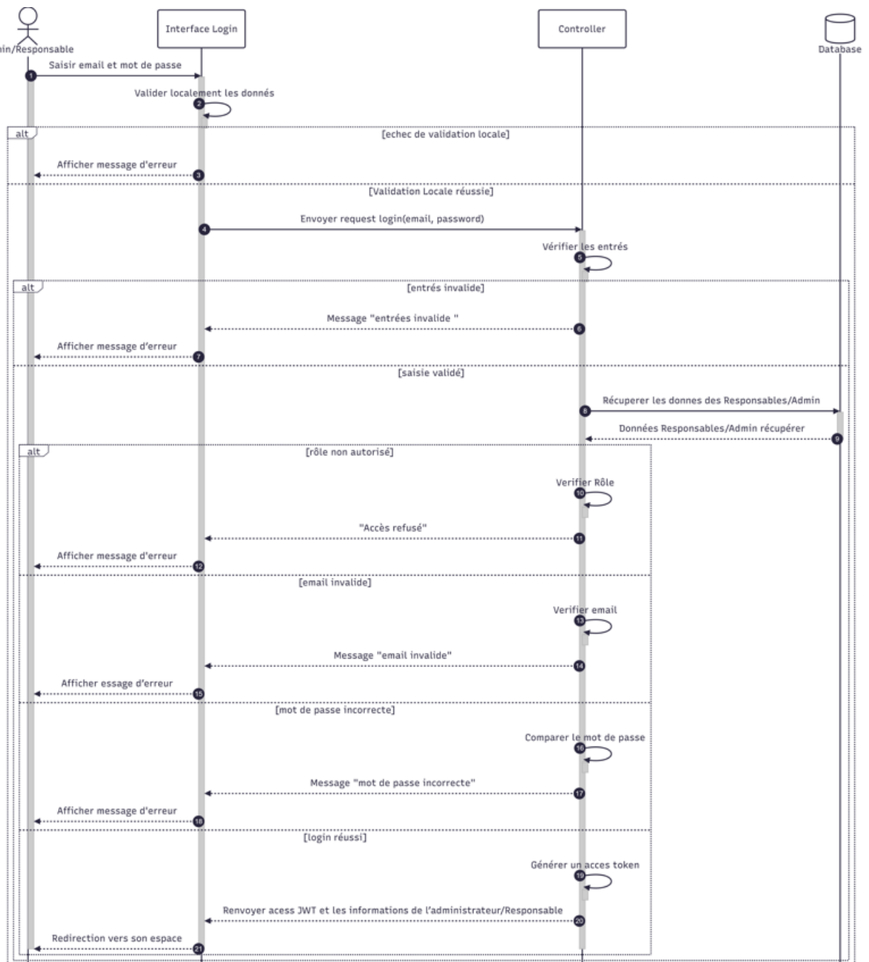
FIGURE 4.7 – Diagramme de séquence «Login -Responsables et Administrateurs»
