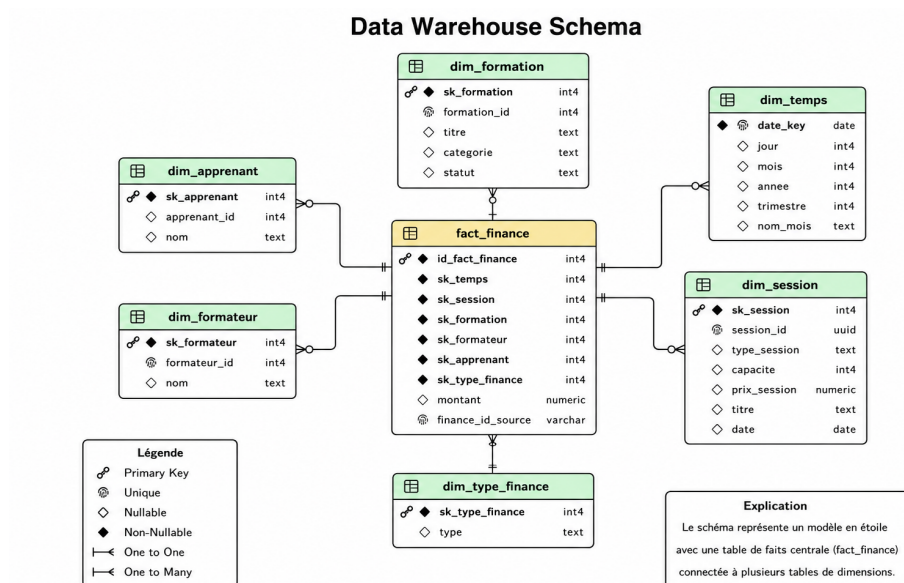
FIGURE 6.3 – Schéma en Étoile
