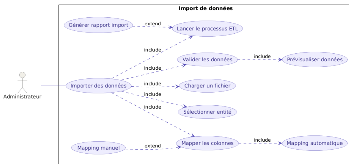
FIGURE 5.30 – Diagramme de cas d'utilisation « Importer des données »
