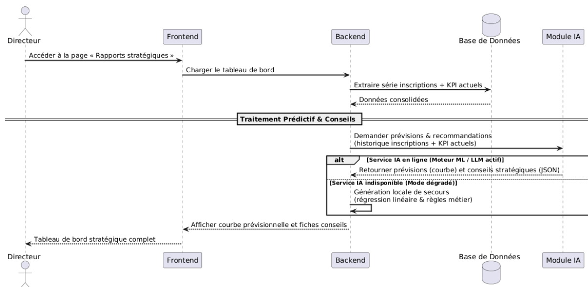
FIGURE 6.20 – Diagramme de séquence « Rapports stratégiques »
