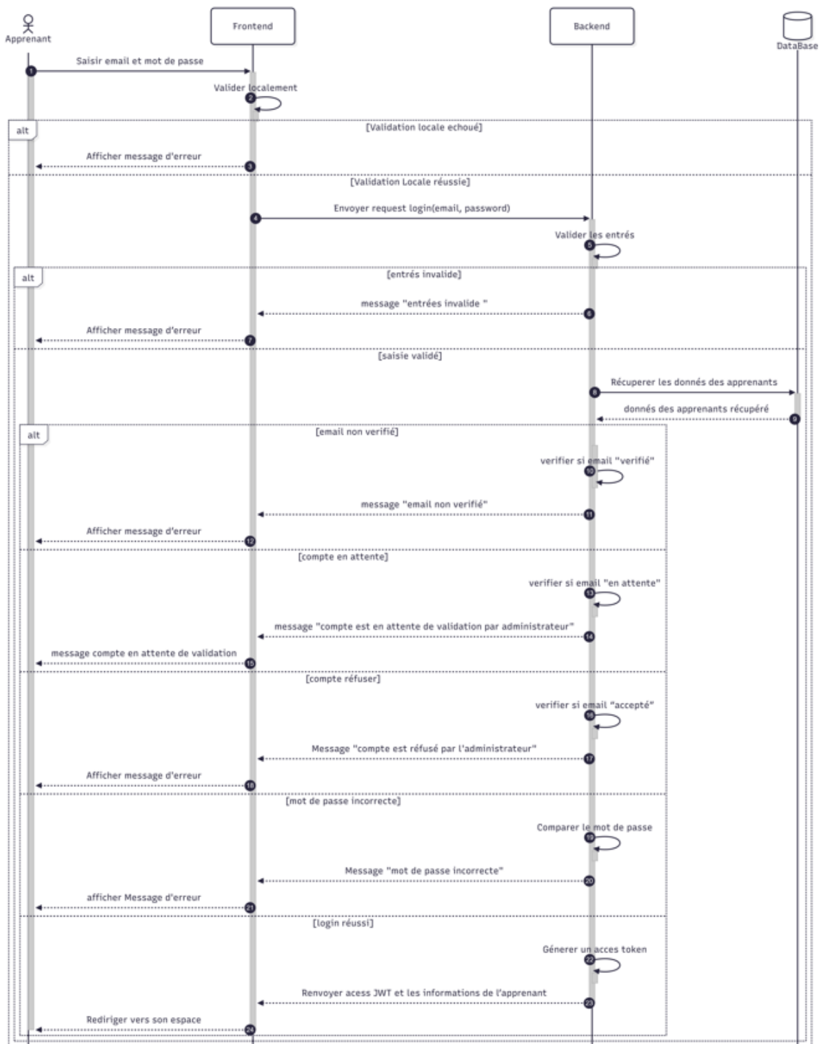
FIGURE 4.6 – Diagramme de séquence «Login - Apprenant»
