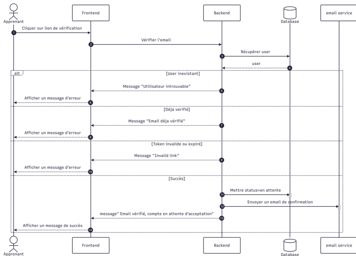
FIGURE 4.5 – Diagramme de séquence «Vérification de l'adresse email»
