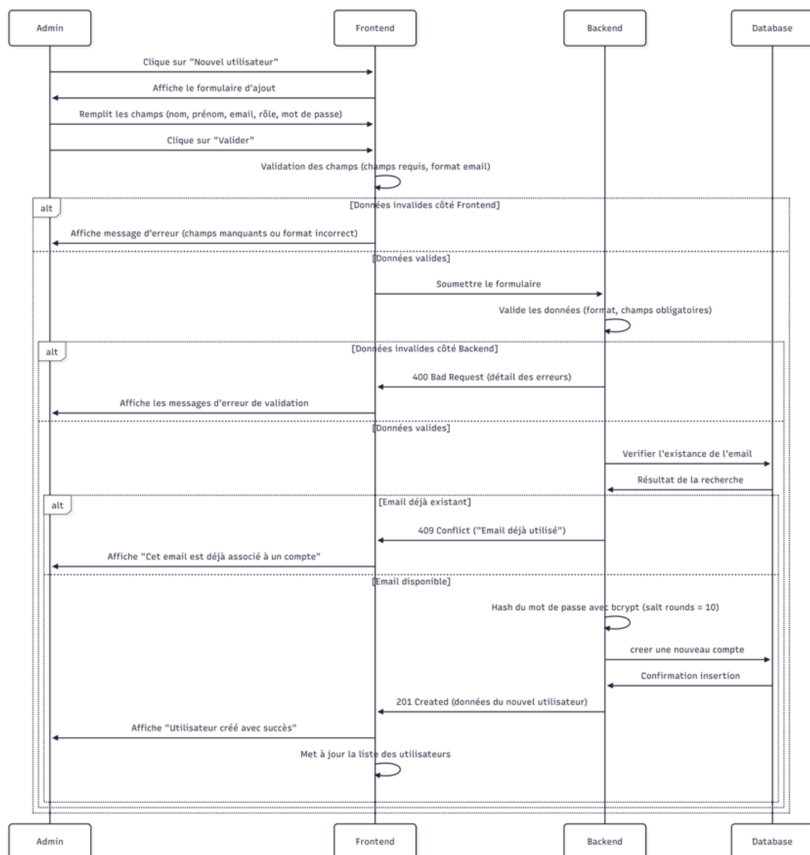
FIGURE 4.32 – Diagramme de séquence «Ajouter un utilisateur»
