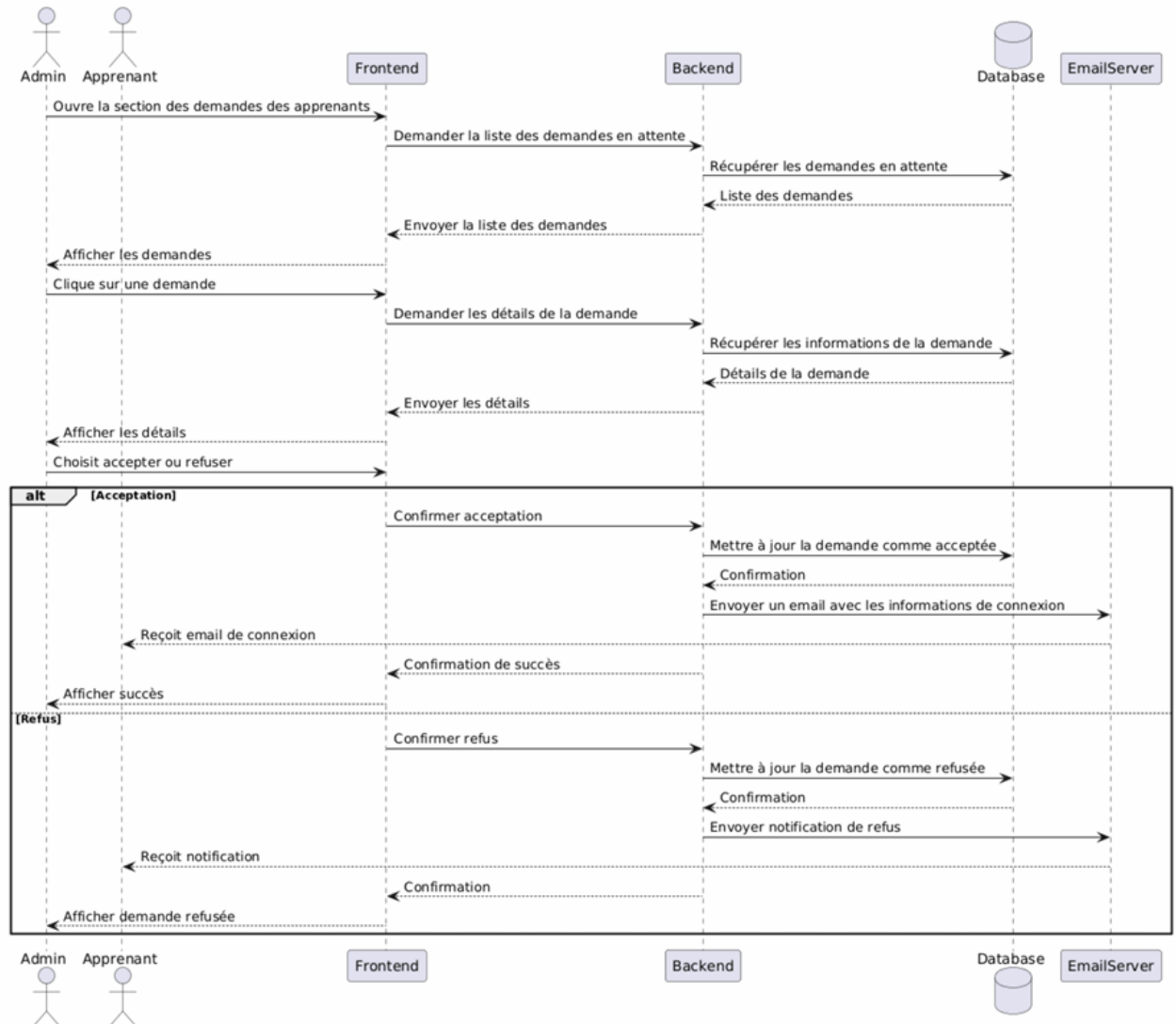
FIGURE 4.34 – Diagramme de séquence «Gestion des demandes des apprenants»
