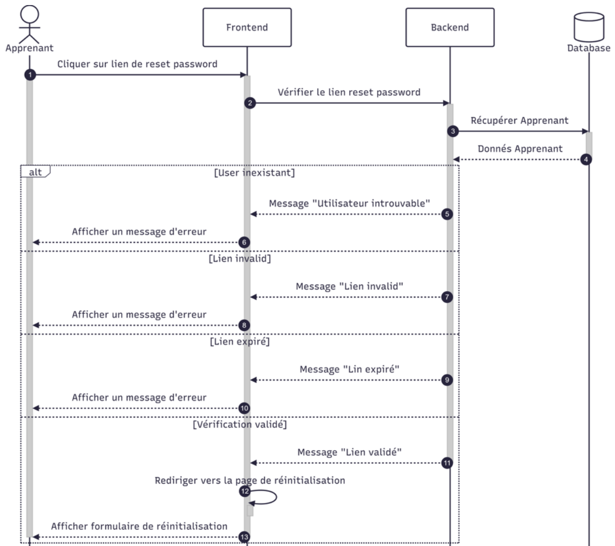
FIGURE 4.8 – Diagramme de séquence «Vérification du lien de réinitialisation»
