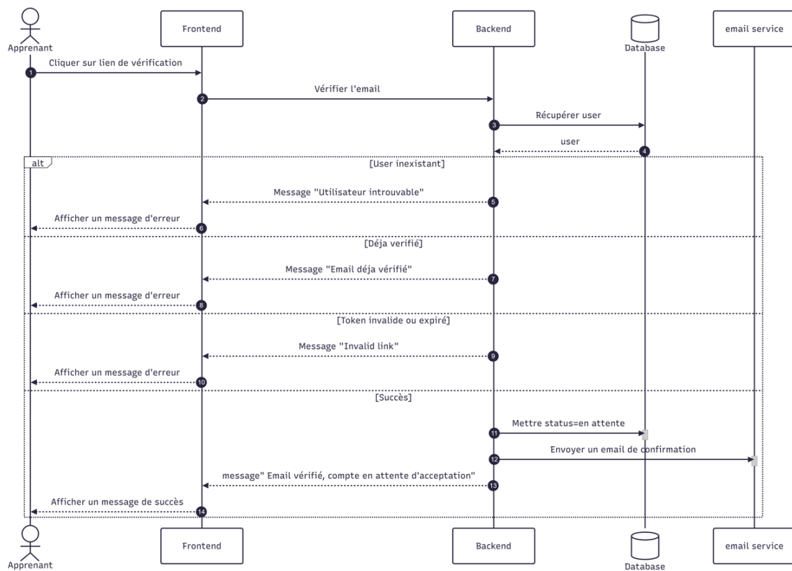
FIGURE 4.4 – Diagramme de séquence «Vérification de l'adresse email»
