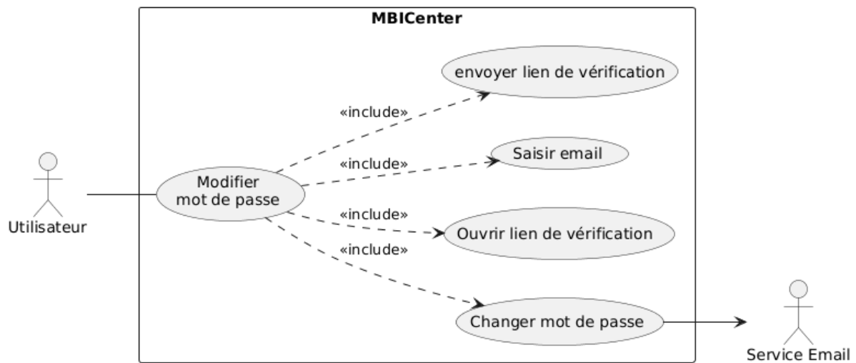
FIGURE 4.2 – Diagramme de cas d'utilisation "modification du mot de passe"
