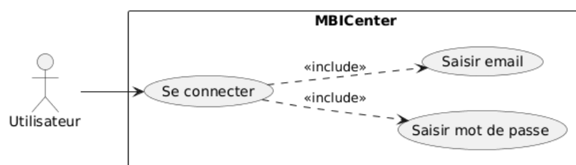
FIGURE 4.1 – Diagramme de cas d'utilisation "authentification"
