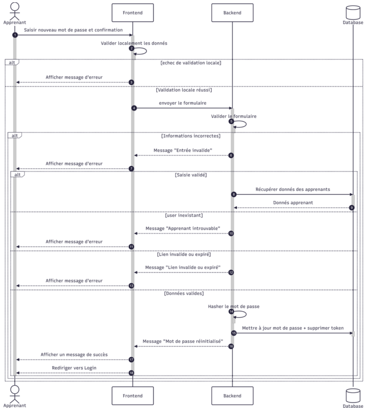
FIGURE 4.9 – Diagramme de séquence «Réinitialisation du mot de passe»
