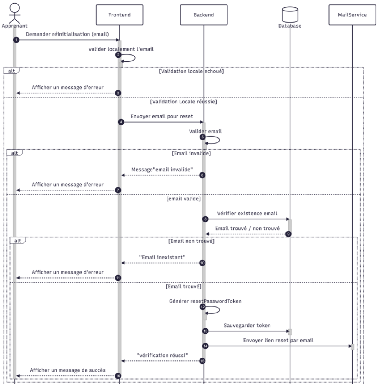
FIGURE 4.7 – Diagramme de séquence «Mot de passe oublié»
