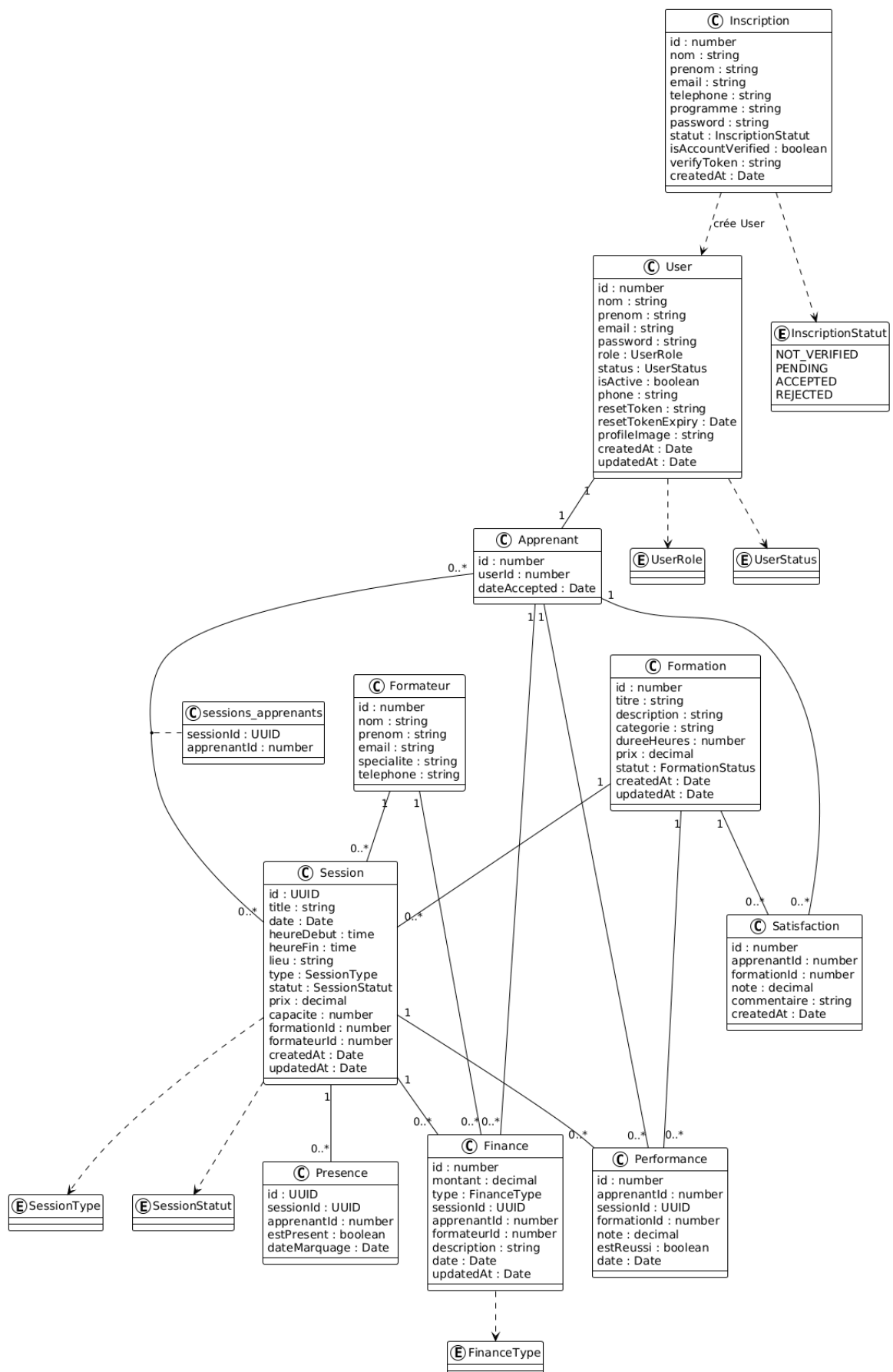
FIGURE 3.16 – Diagramme de classe
