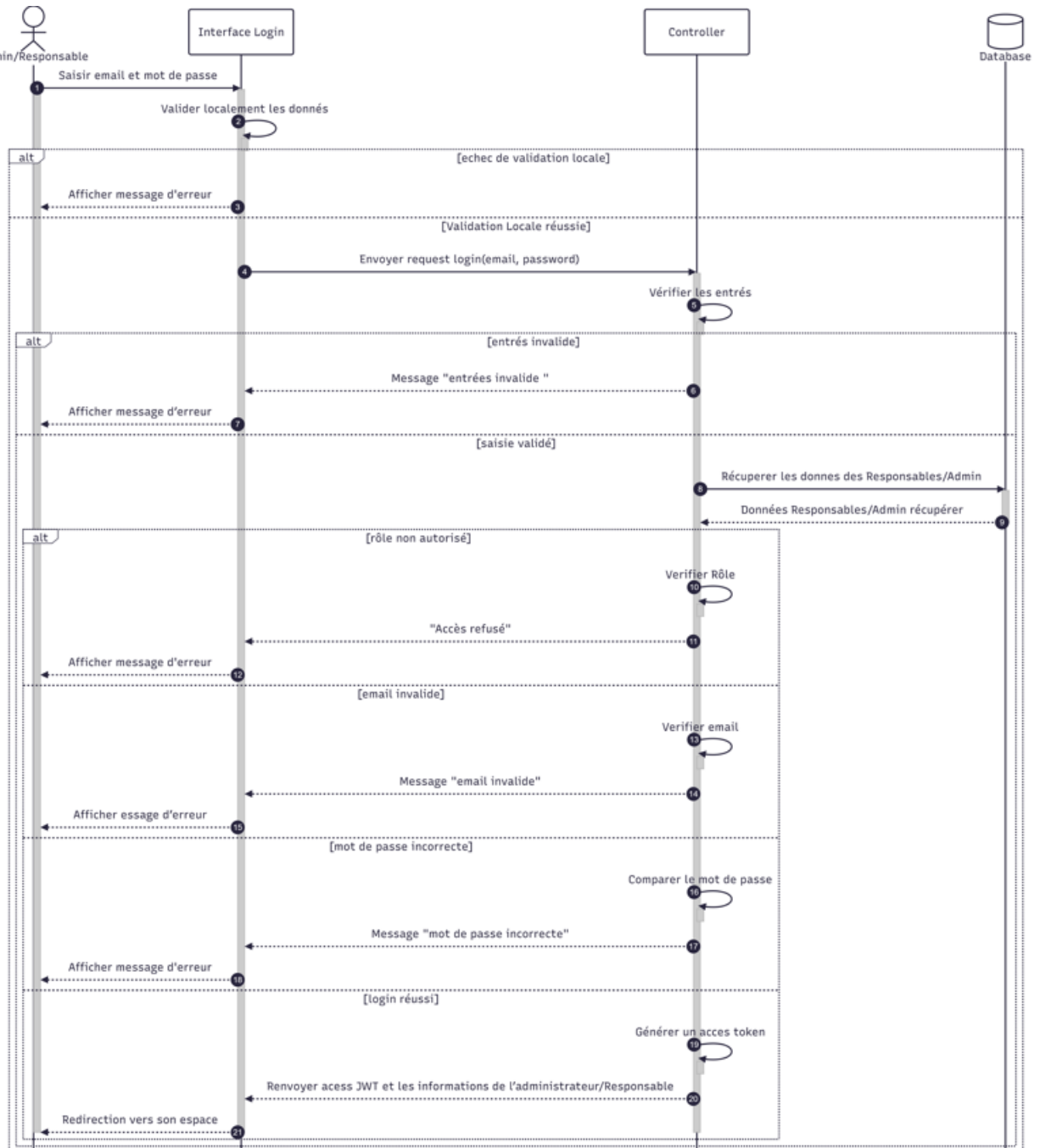
FIGURE 4.6 – Diagramme de séquence «Login -Responsables et Administrateurs»
