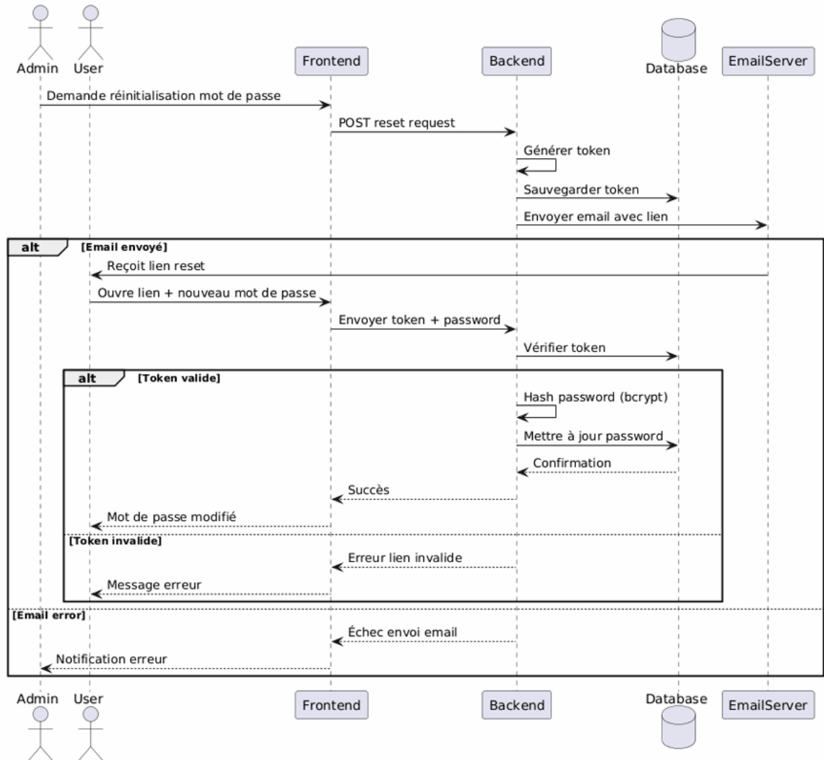
FIGURE 4.33 – Diagramme de séquence «Réinitialisation du mot de passe»
