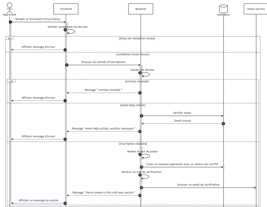
FIGURE 4.3 – Diagramme de séquence «Inscription de l'apprenant»
