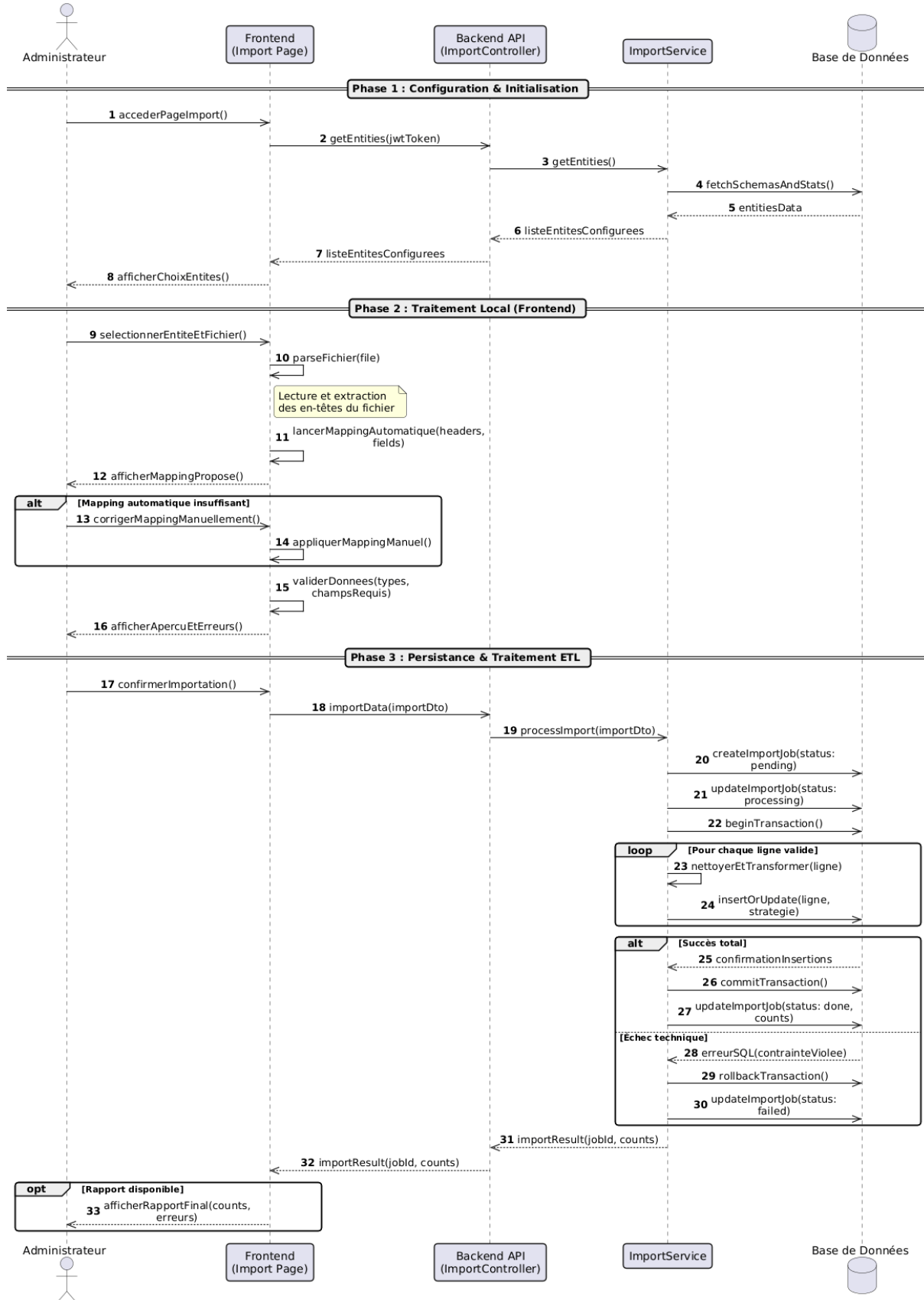
FIGURE 5.2 – Diagramme de séquence « Importer des données »
