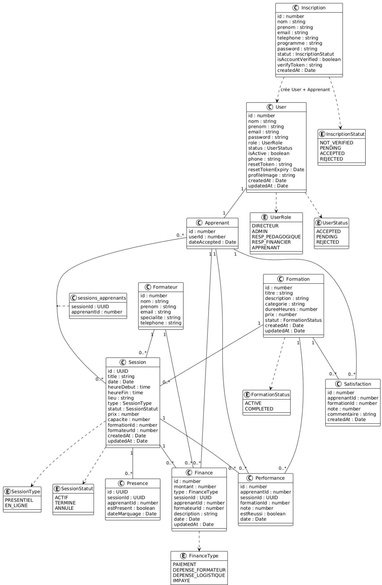
FIGURE 3.16 – Diagramme de classe
