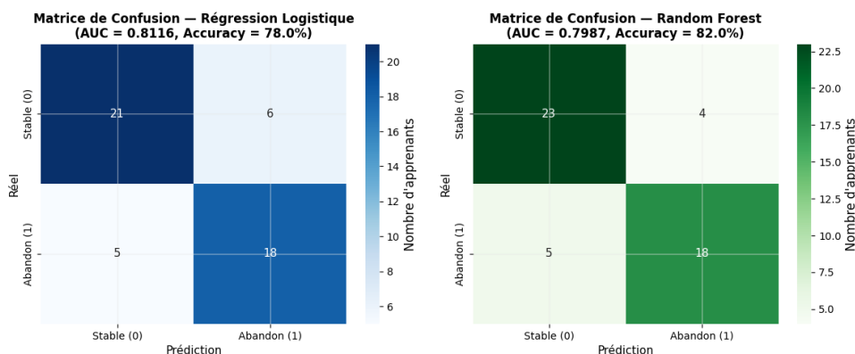
FIGURE 6.22 – Matrices de confusion — Prédiction du risque d'abandon
