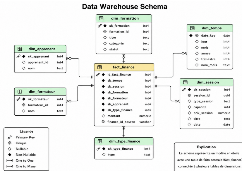
FIGURE 6.3 – Schéma en Étoile
