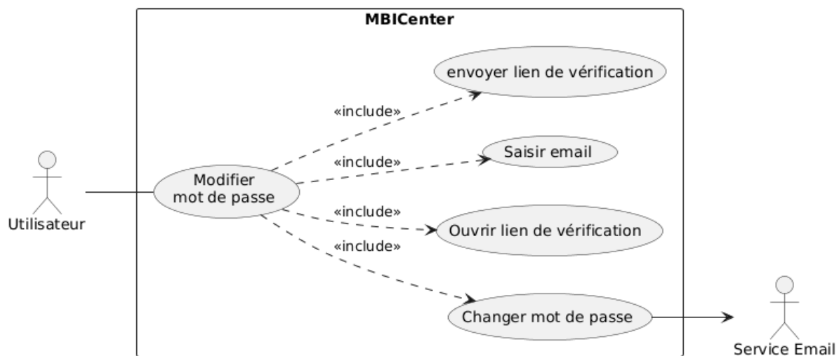
FIGURE 4.3 – Diagramme de cas d'utilisation "modification du mot de passe"
