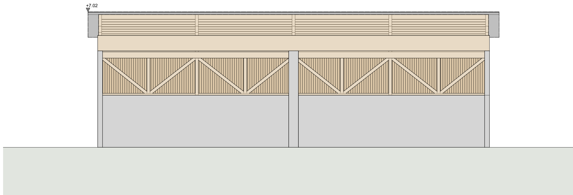
ANSICHT SÜD-WEST
