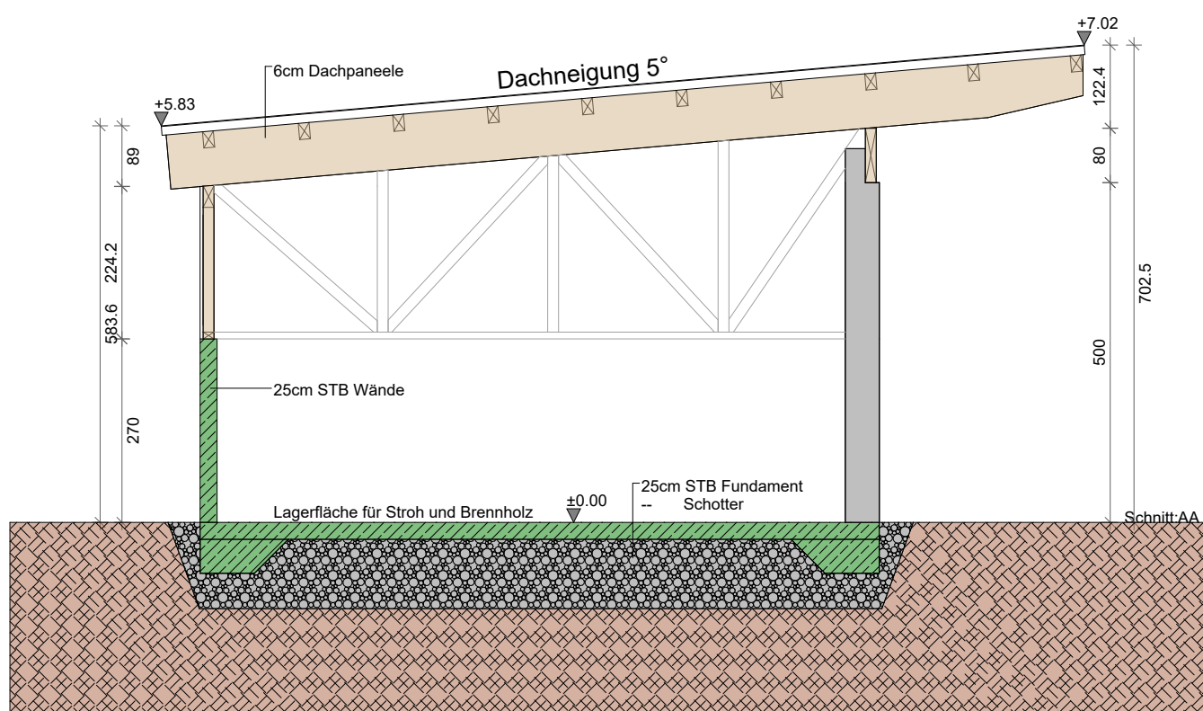
SCHNITT A-A
