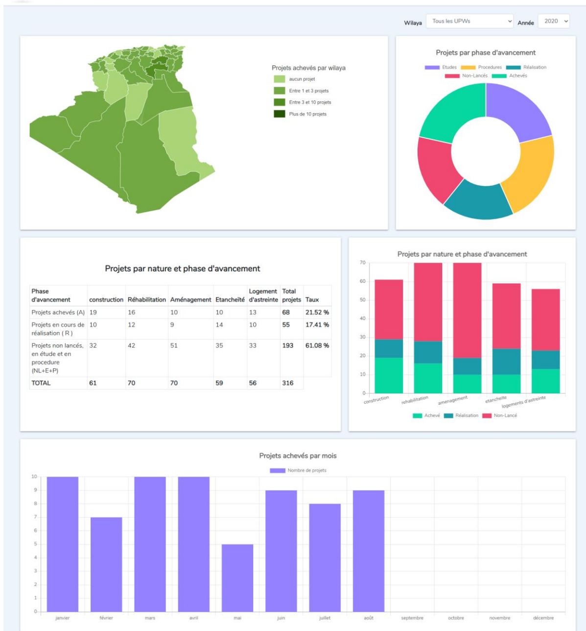
Figure 2. Page d'accueil.
