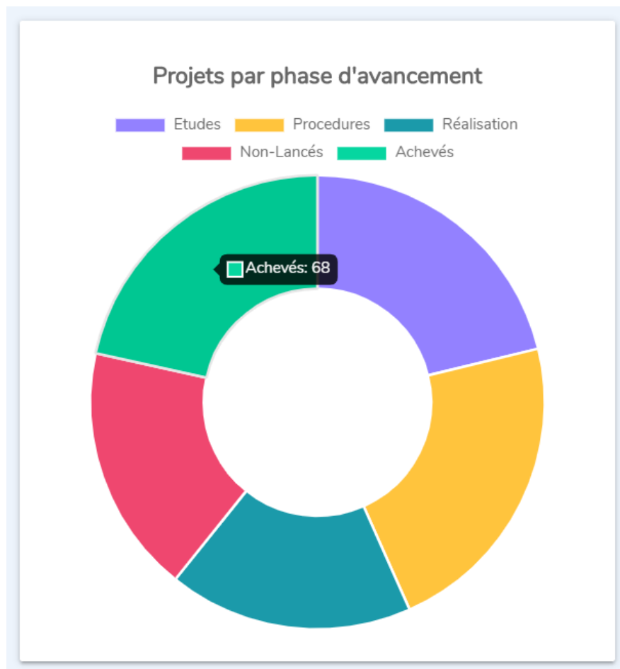
Figure 4. Diagramme circulaire.
