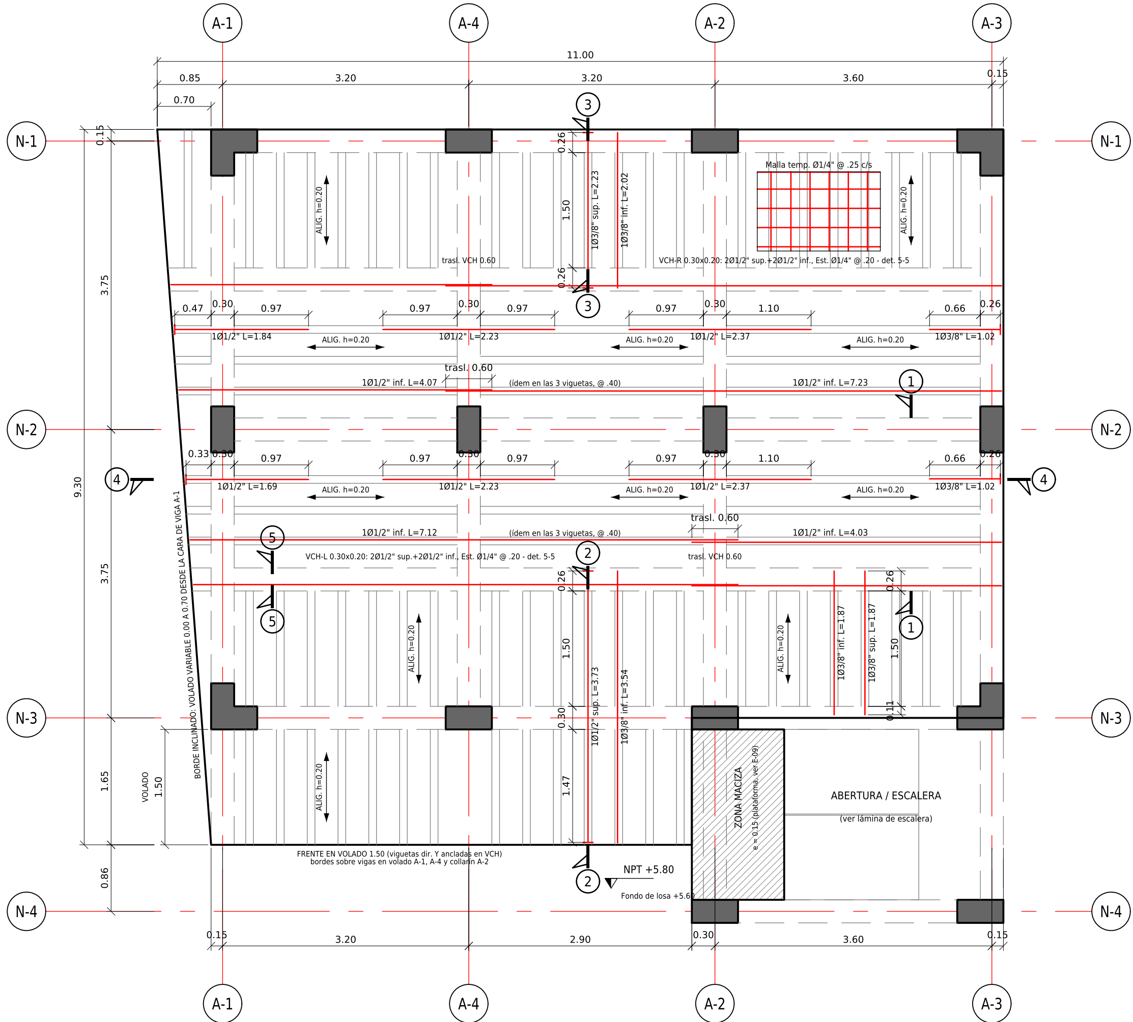
PLANTA DE LOSA ALIGERADA - NIVEL 3 (NPT +5.80)
