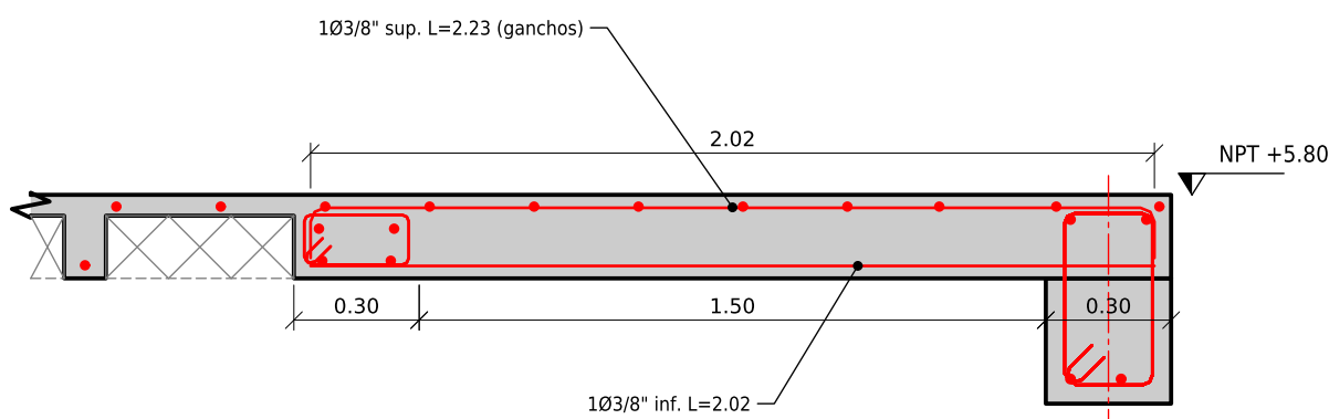
CORTE 3-3 BORDE N-1 Y VCH
