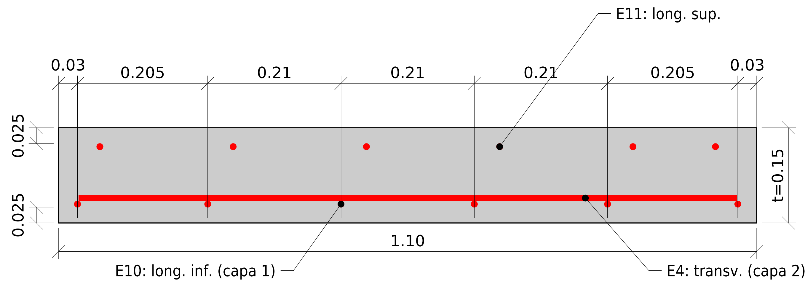
SECCIÓN TÍPICA DE TRAMO (perpendicular a la losa)
