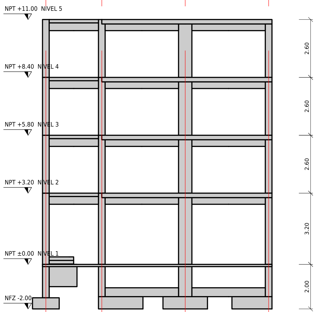
CORTE GENERAL EJE A-2
