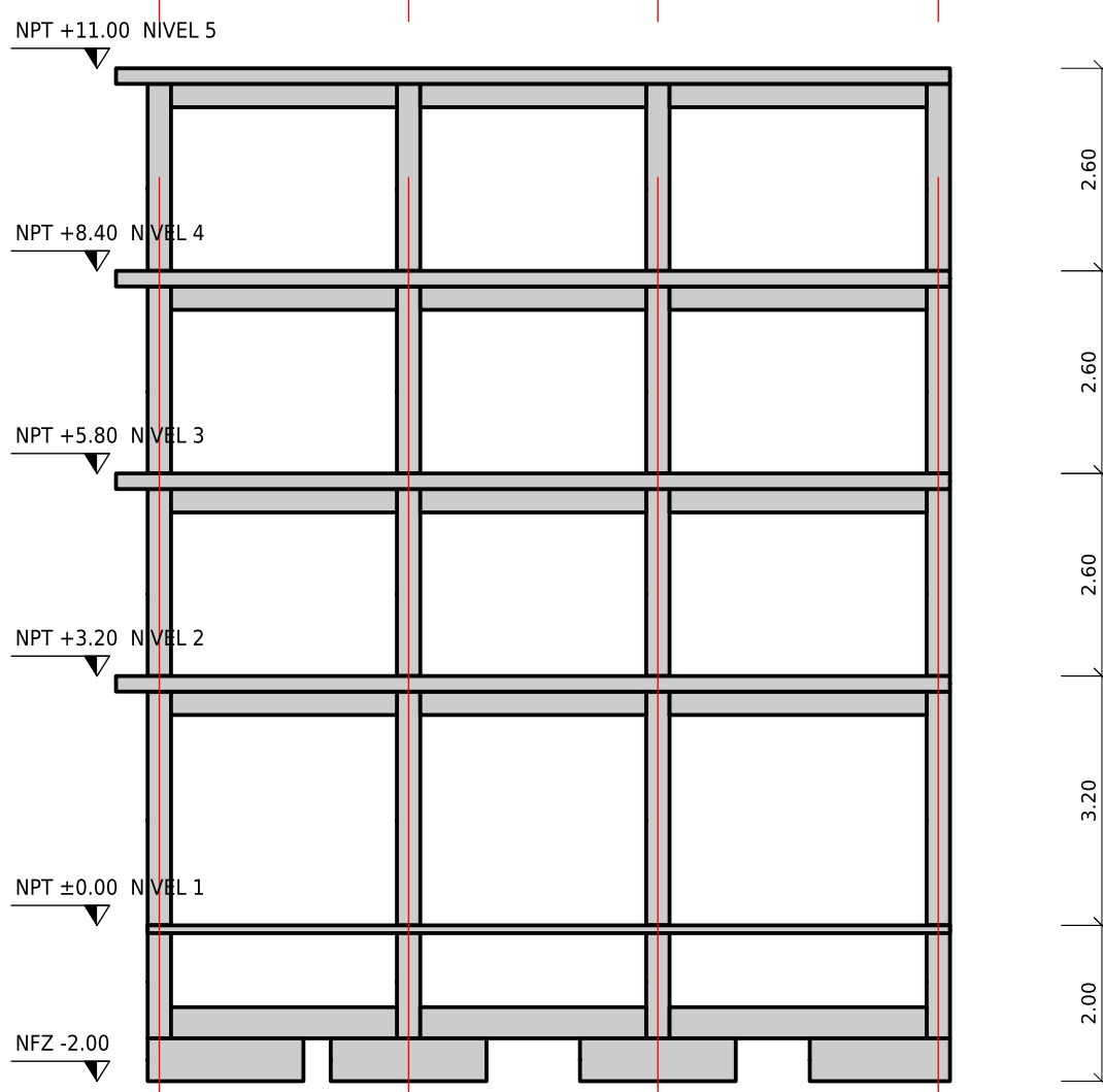
CORTE GENERAL EJE N-2
