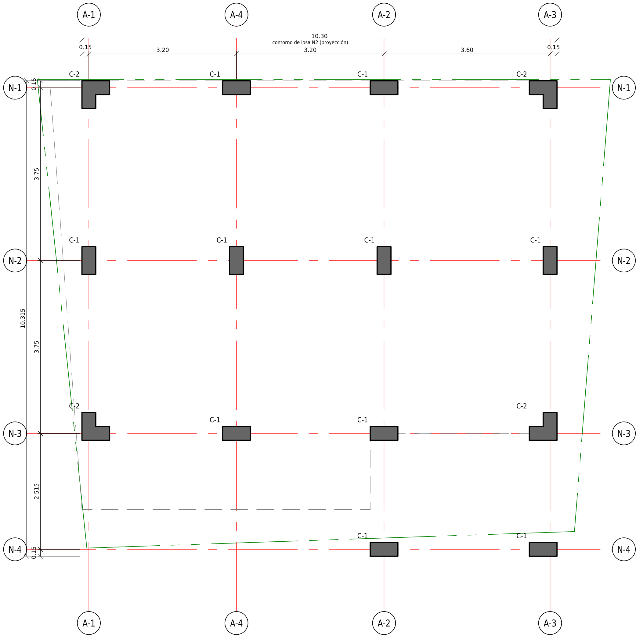
PLANTA DE COLUMNAS Y REPLANTEO (N1 a N5)
