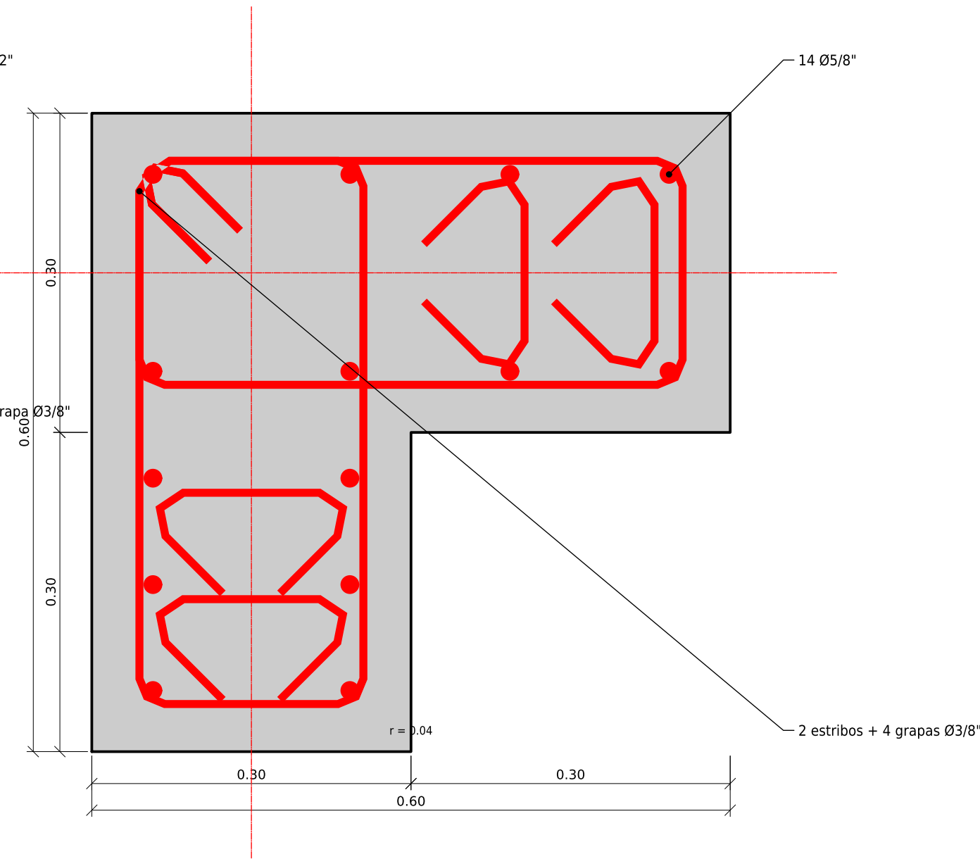
SECCIÓN C-2 ESC. 1:5 (corte en zona central)
