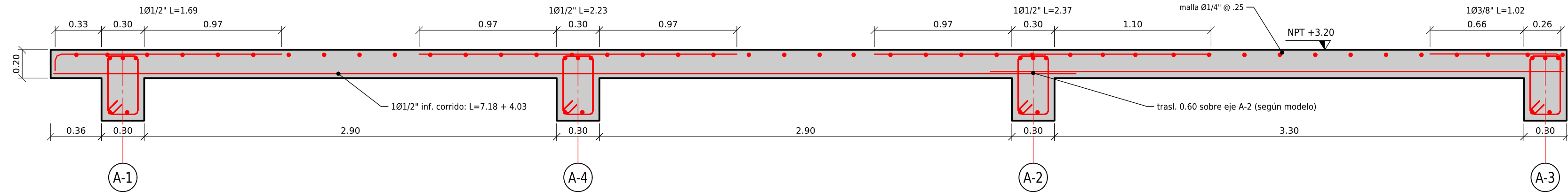
CORTE 4-4 LONGITUDINAL DE VIGUETA (dir. X)
