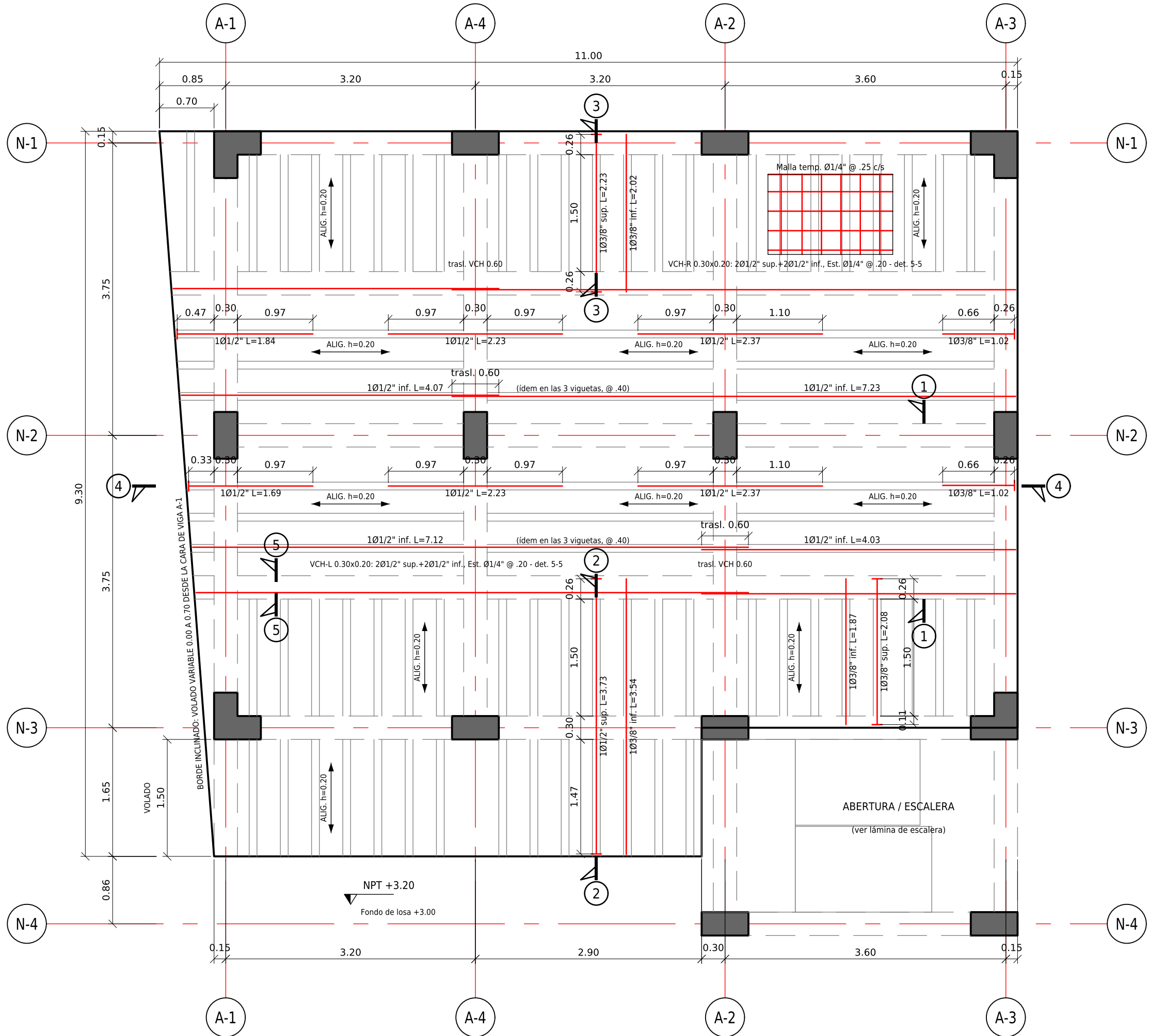
PLANTA DE LOSA ALIGERADA - NIVEL 2 (NPT +3.20)
