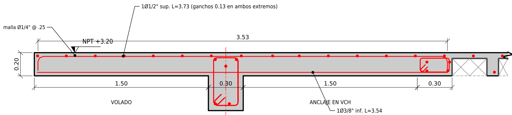
CORTE 2-2 VOLADO LADO N-4 Y VCH
