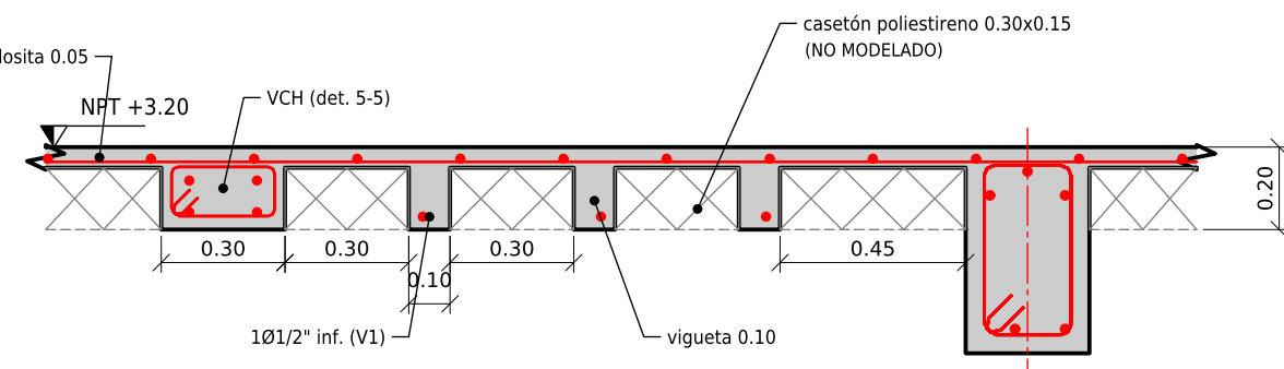
CORTE 1-1 ALIGERADO TÍPICO
