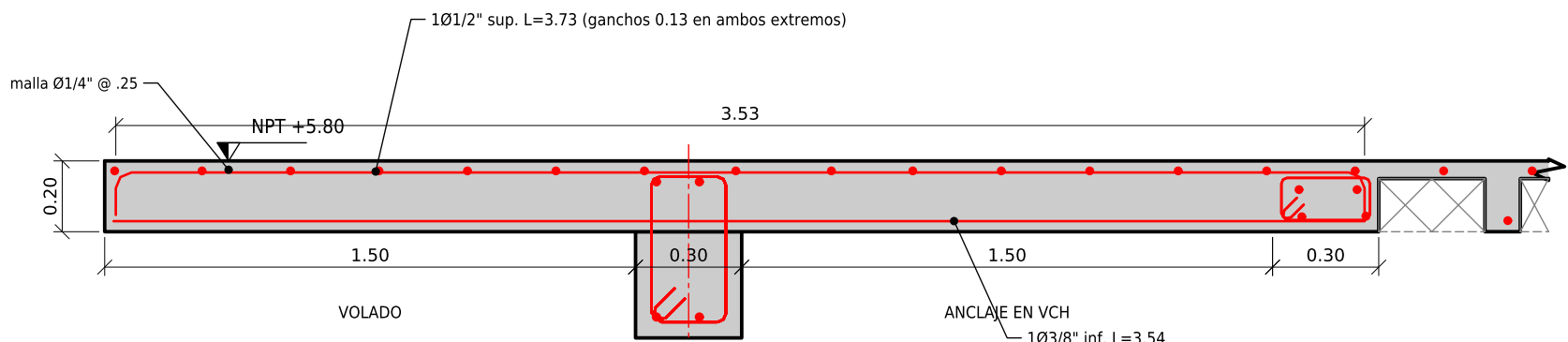
CORTE 2-2 VOLADO LADO N-4 Y VCH
