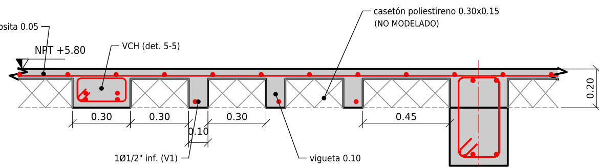
CORTE 1-1 ALIGERADO TÍPICO
