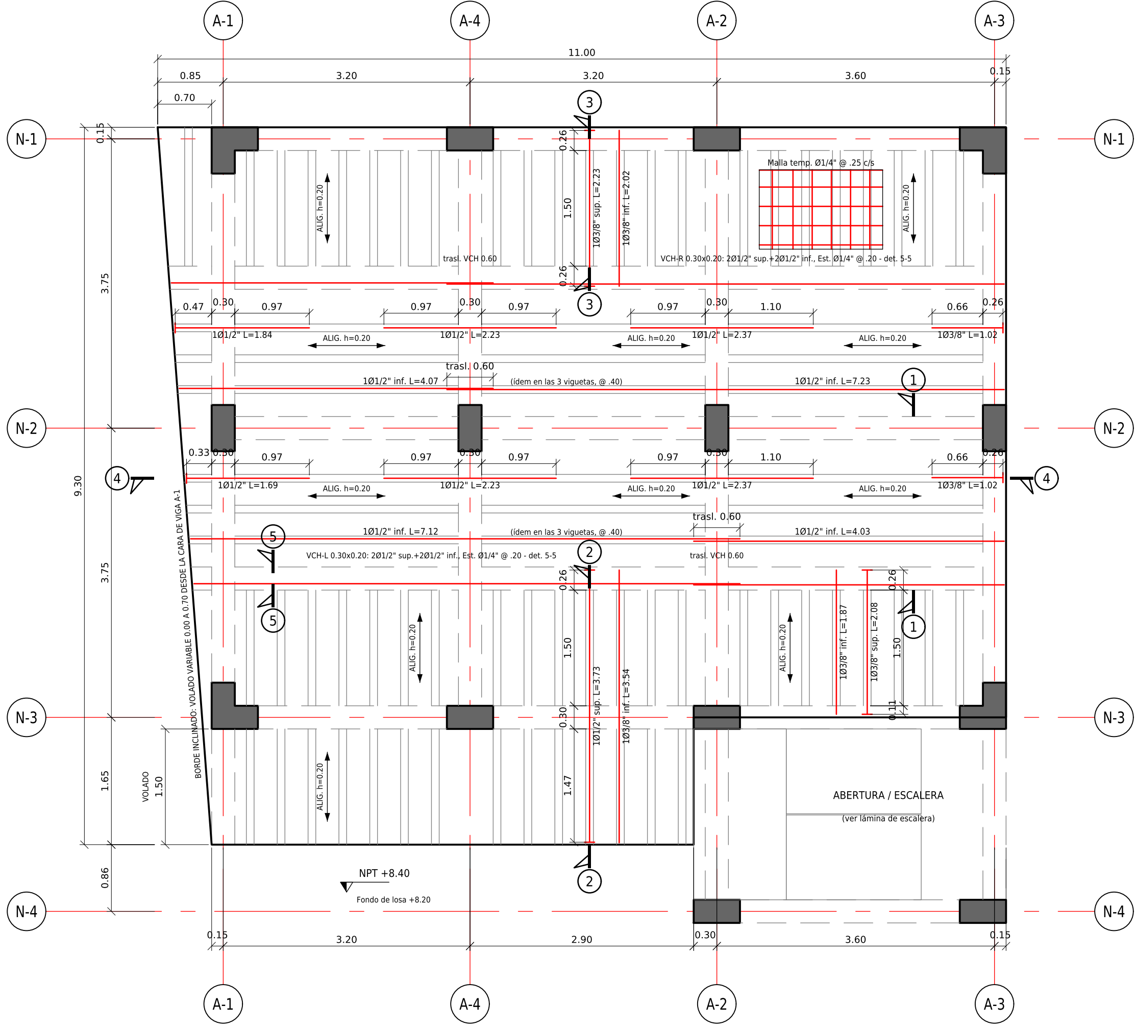
PLANTA DE LOSA ALIGERADA - NIVEL 4 (NPT +8.40)
