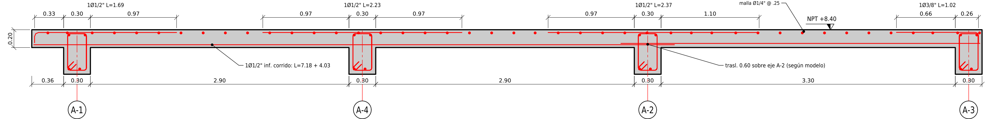
CORTE 4-4 LONGITUDINAL DE VIGUETA (dir. X)
