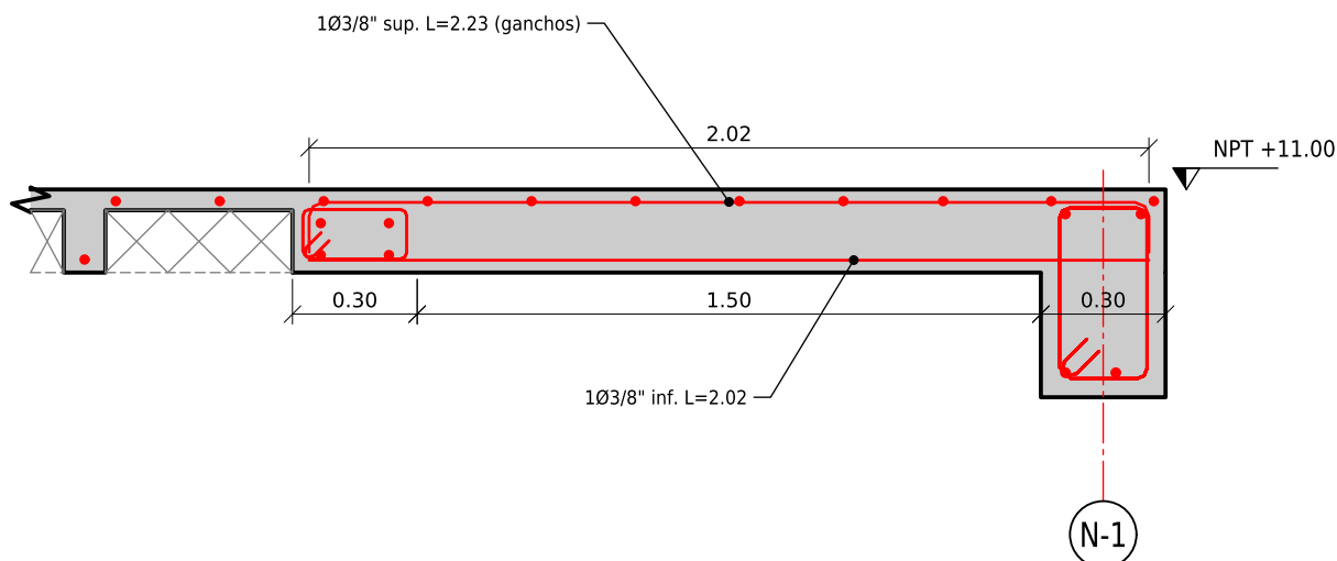
CORTE 3-3 BORDE N-1 Y VCH
