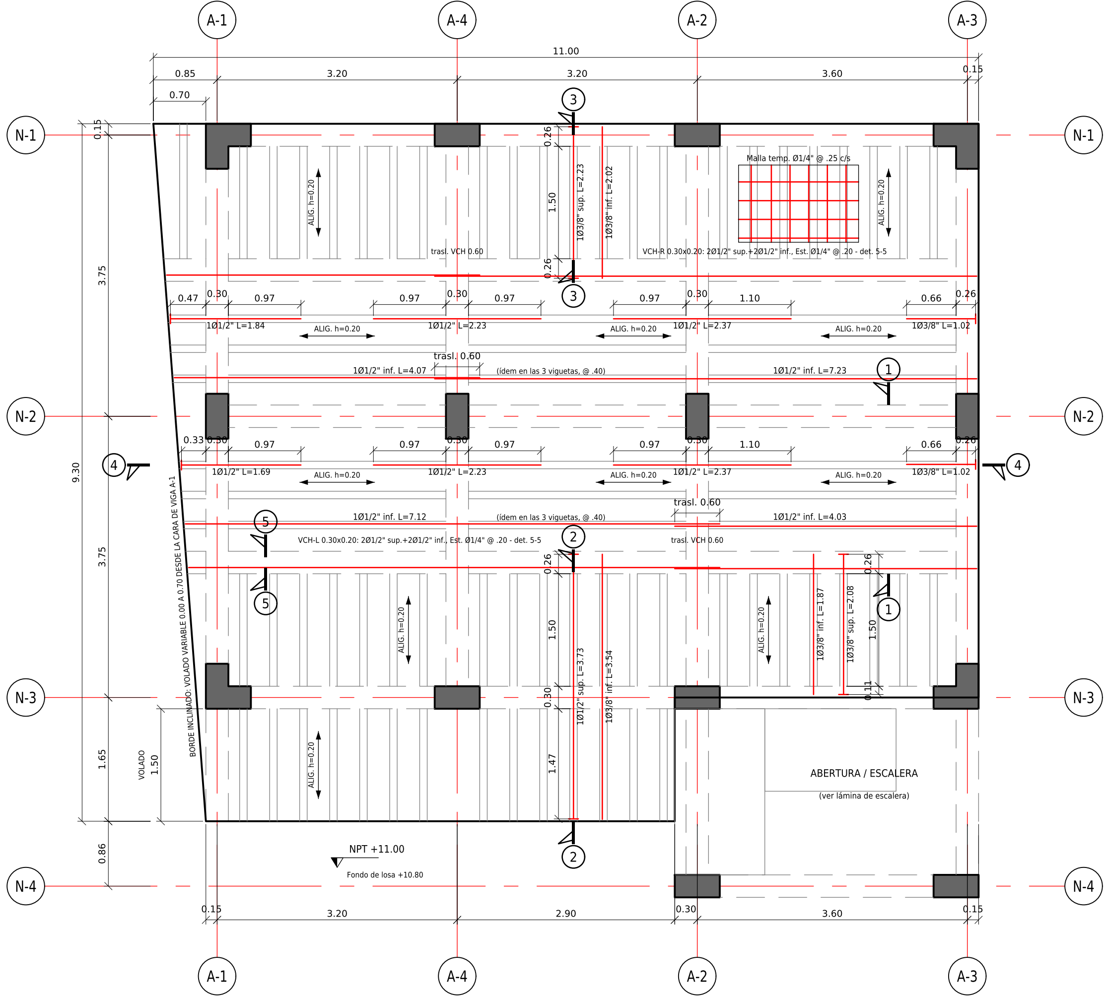
PLANTA DE LOSA ALIGERADA - NIVEL 5 (NPT +11.00)
