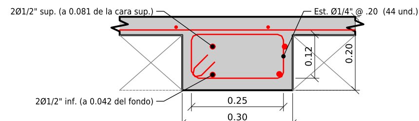
DETALLE 5-5 VIGA CHATA VCH
