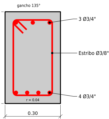
VE-3 0.30 x 0.50
