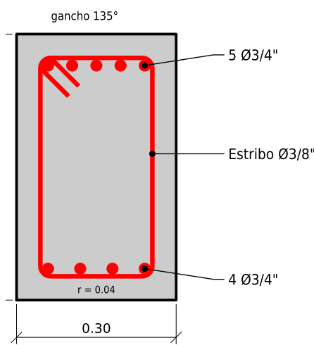
VE-5 0.30 x 0.50
