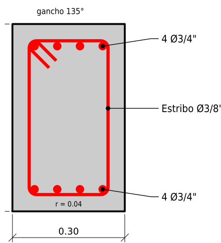
VE-4 0.30 x 0.50
