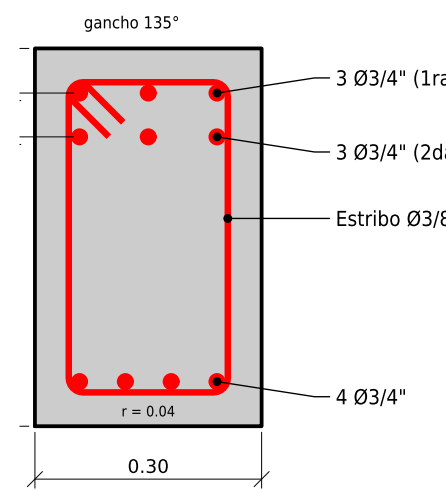
VE-6 0.30 x 0.50
